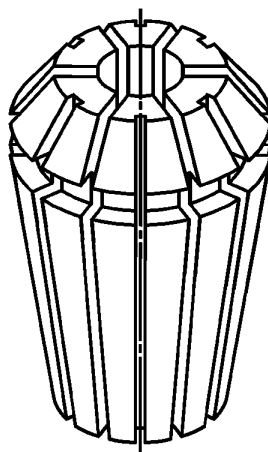
Рисунок 9д) — Зажимная цанга для крепления оправки с закрепленным на ней инструментом
