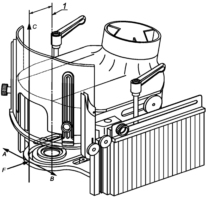
1 — ось шпинделя
