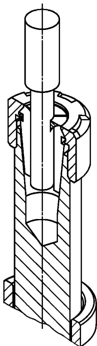
Рисунок 9с) — Пример применения сменных прижимных втулок-вкладышей для крепления оправки с закрепленным на ней инструментом
