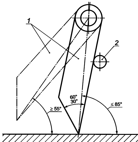
1 — противовыбрасывающий элемент; 2 — ограничительный упор
