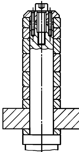
Рисунок 9б) — Пример применения винта, двух штифтов и специального фланца
