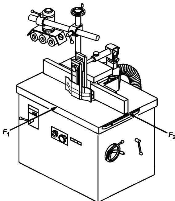
Рисунок С.1 — Испытание на устойчивость передвижных станков
