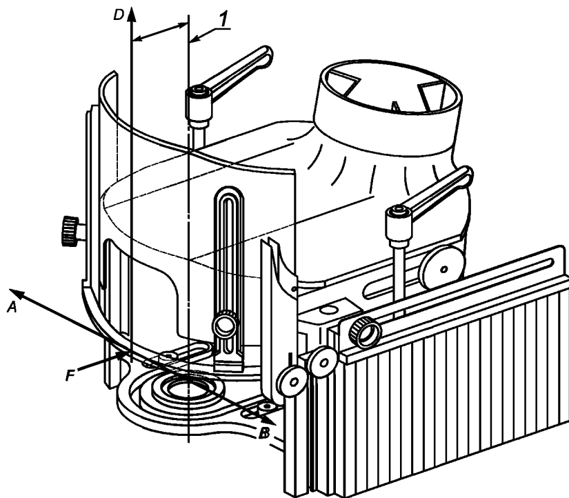
1 — ось шпинделя
