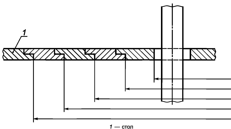
Рисунок 15 — Кольца стола
