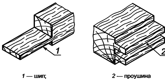
Рисунок 3 — Пример обработанной заготовки с шипом/проушиной
