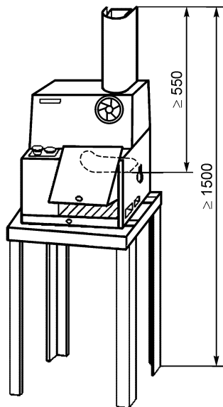
Рисунок 4 — Безопасные расстояния
