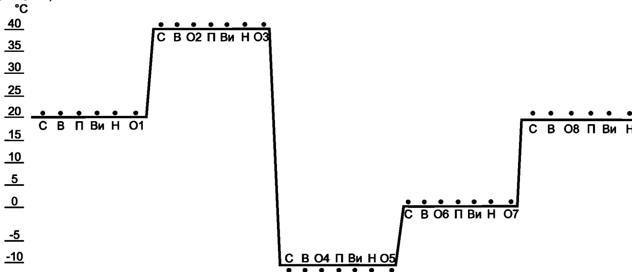
Рисунок 11 — Предлагаемая последовательность испытаний по A.5.3.1, совмещенных с A.5.3.2 (температурные испытания в диапазоне от минус 10 °C до плюс 40 °C)
