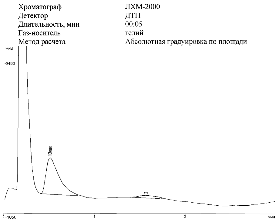
Рисунок М.4 – Типичная хроматограмма пробы масла
