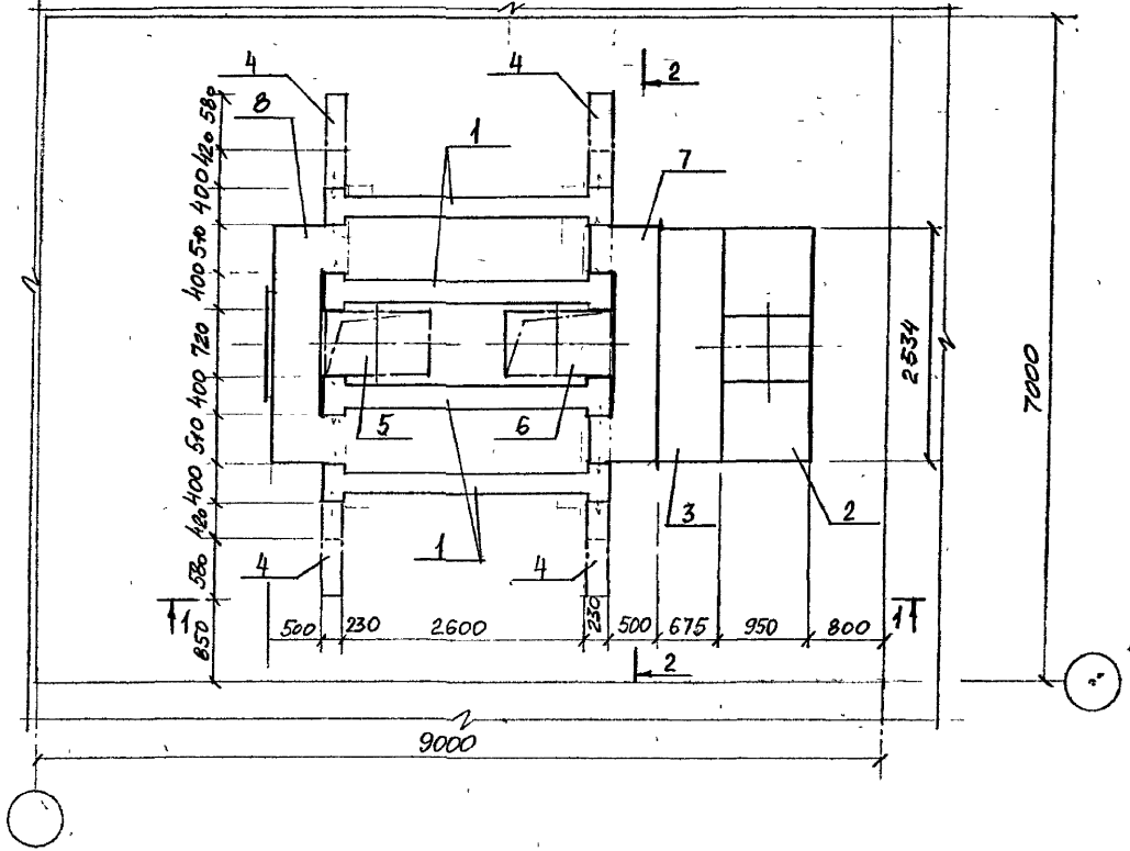
ПЛАН
