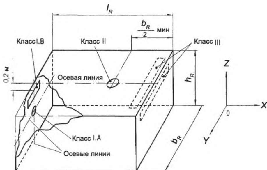
Рисунок 6 - Монтаж воздухораспределительных устройств на второй испытательной установке
