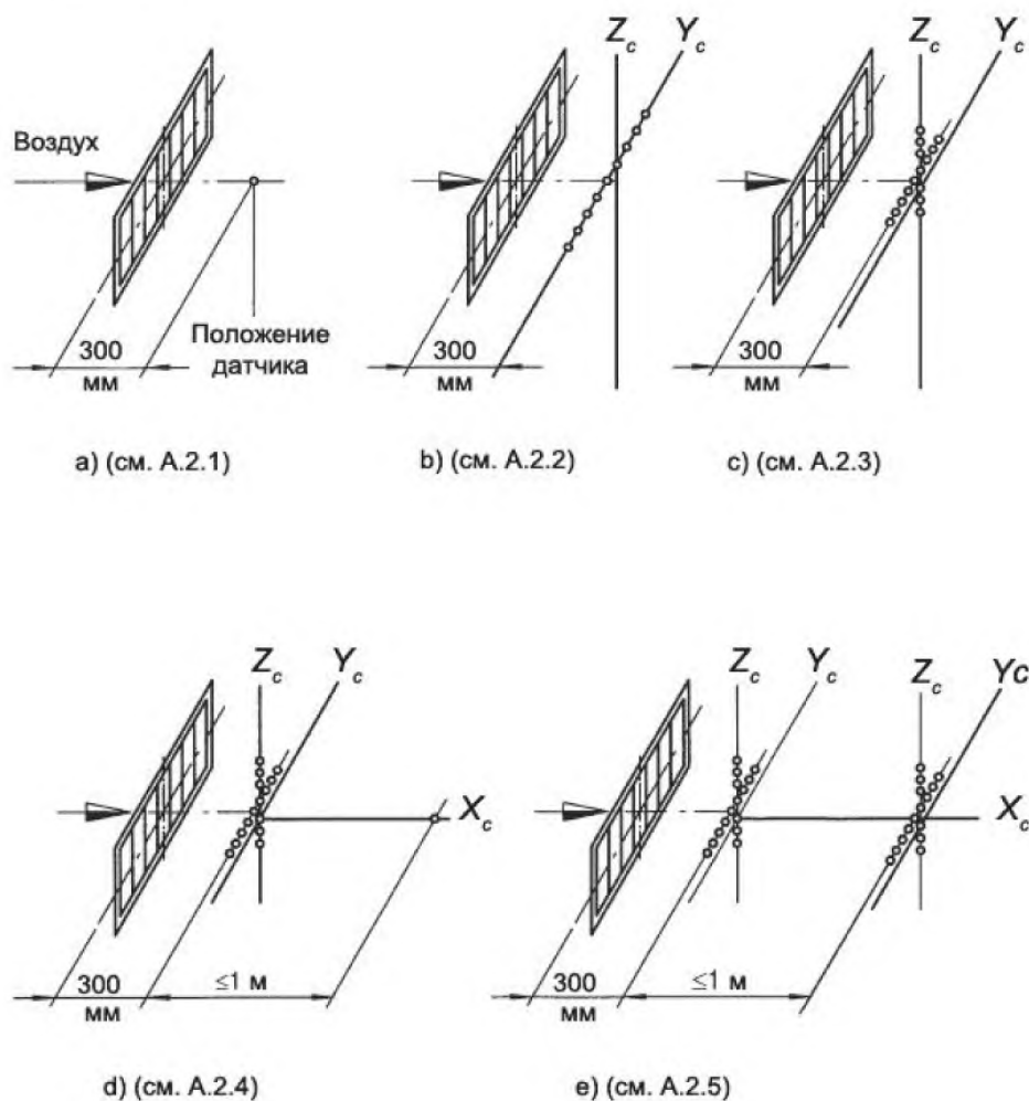
Рисунок А.1 - Определение координат максимальной скорости
