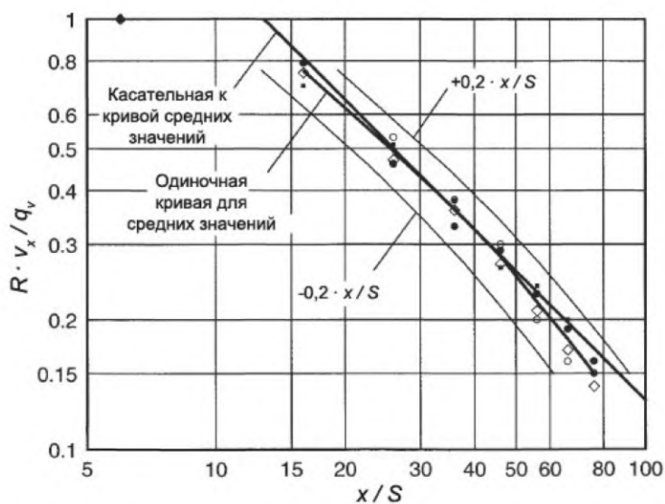
Рисунок 8 - Характерный график для определения дальности
