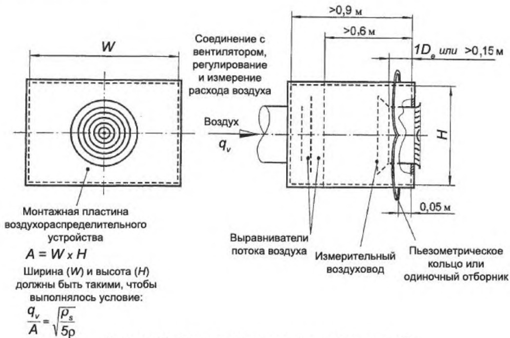
Рисунок 3 - Первая испытательная установка В для приточных воздухоораспределительных устройств
