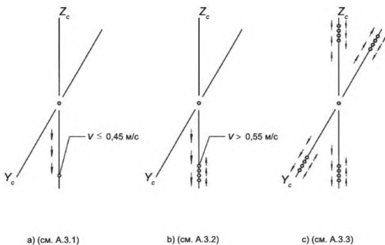
Рисунок А.3 - Определение поверхности постоянных скоростей
