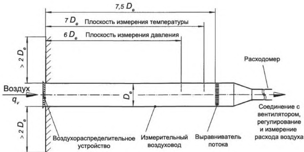
Рисунок 4 - Первая испытательная установка С для вытяжных воздухоораспределительных устройств
