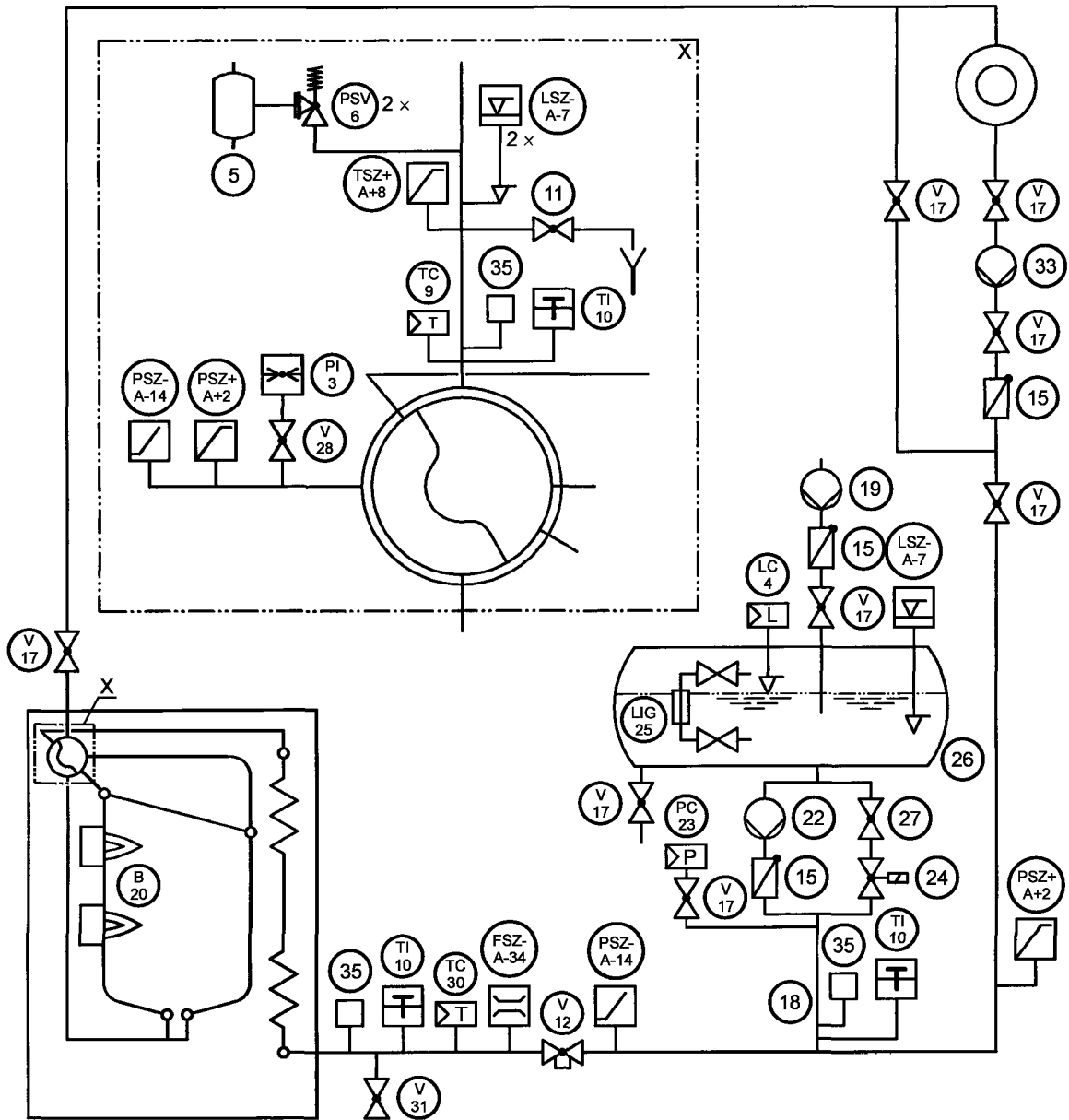
Рисунок В.4-5 — Установки с принудительной циркуляцией, верхней подпиткой воды, с насосами поддержанием давления из внешнего источника
