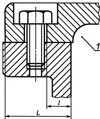
Рисунок 3 — Отверстия на поверхностях плоских соединений (пример 1)
