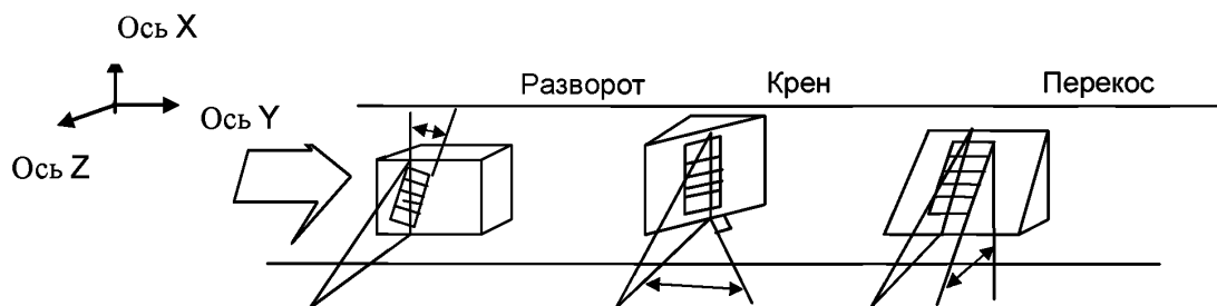
Рисунок 1 – Углы считывания
