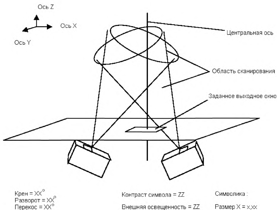
Рисунок В.5 – Диаграмма многооконого сканера
