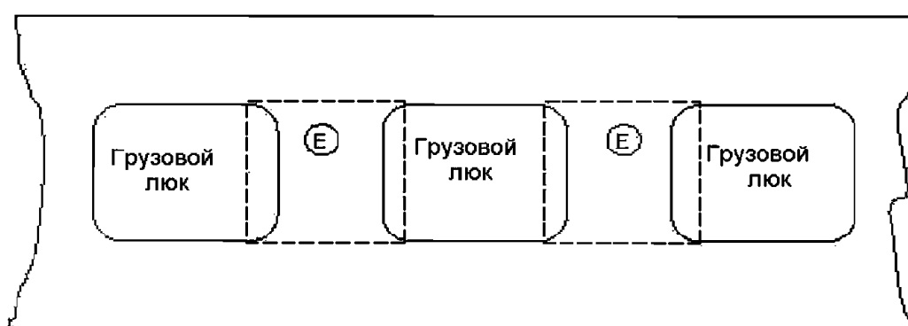
Рис. 6.2.3.2-2 Районы A, C, D и E детальных освидетельствований навалочных судов
