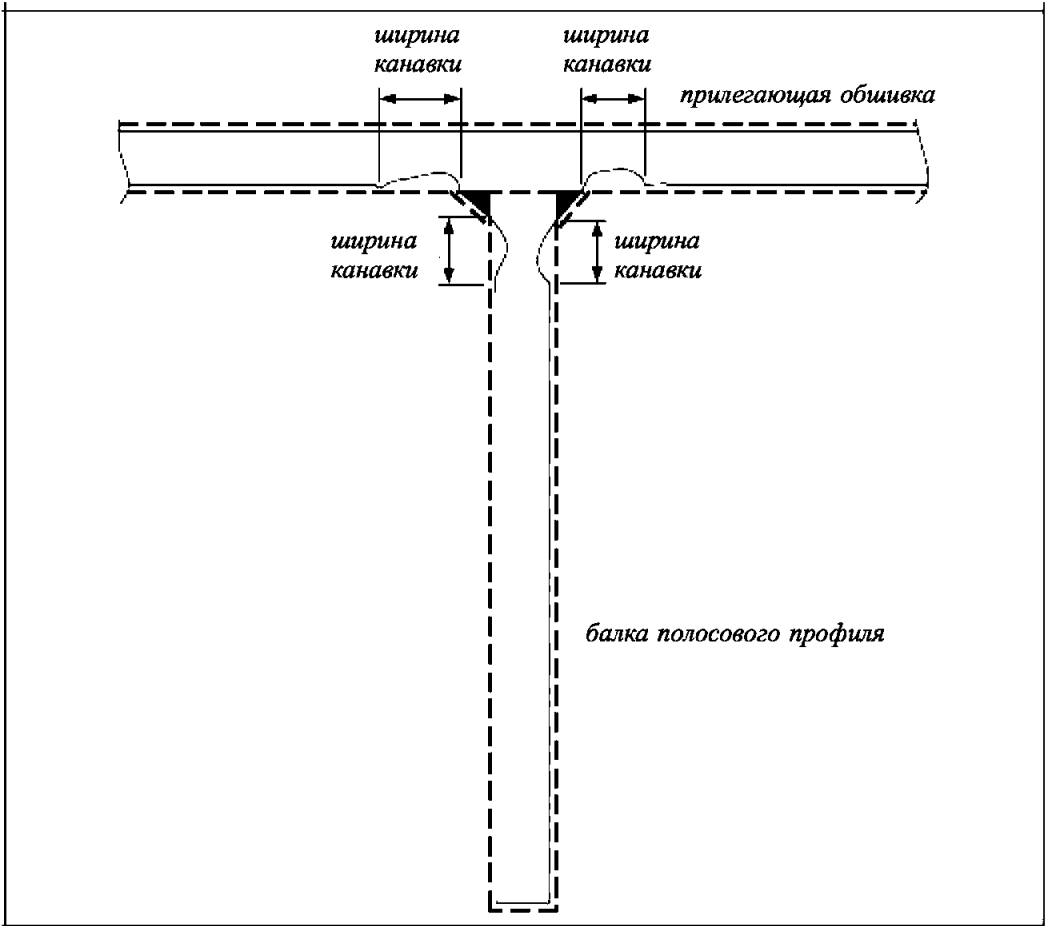
Рис. 1.2.1-4 Канавочный износ
