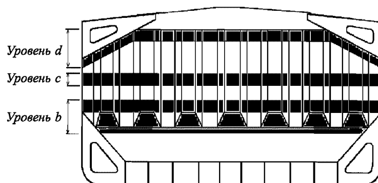
Рис. 5.2.3.2-4 Уровни b, c и d детального освидетельствования поперечных переборок, имеющих верхние и нижние опоры, в грузовых трюмах навалочных судов
