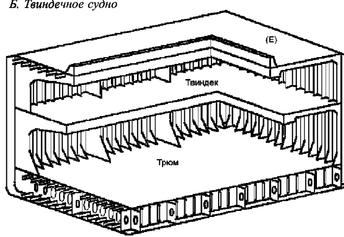
Рис. 7.2.3.2-1 Районы А, В и Е детального освидетельствования судов, предназначенных для перевозки сухих генеральных грузов
