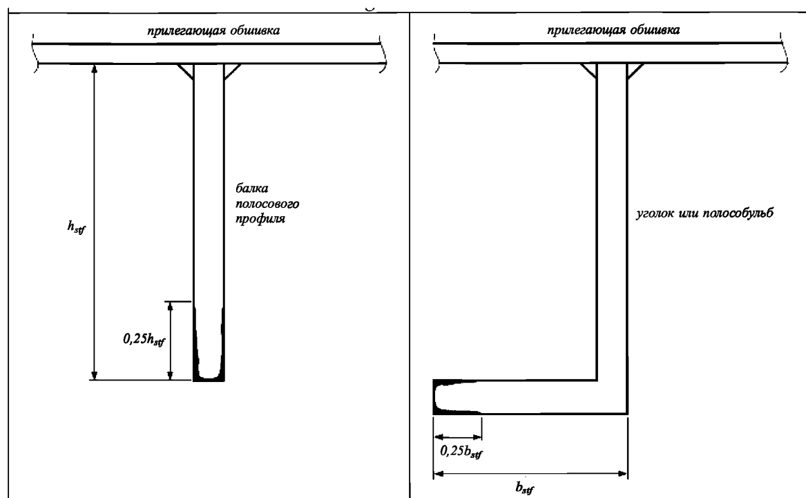
Рис. 1.2.1-5 Коррозия кромок
