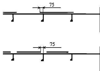
Рис. 5.2.2.4-1 Расположение накладных полос
