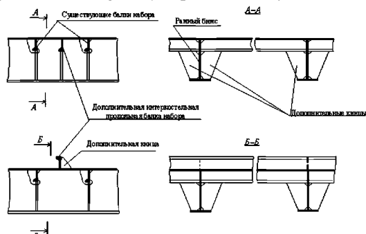
Рис. 5.2.2.4-2 Установка дополнительных балок набора
