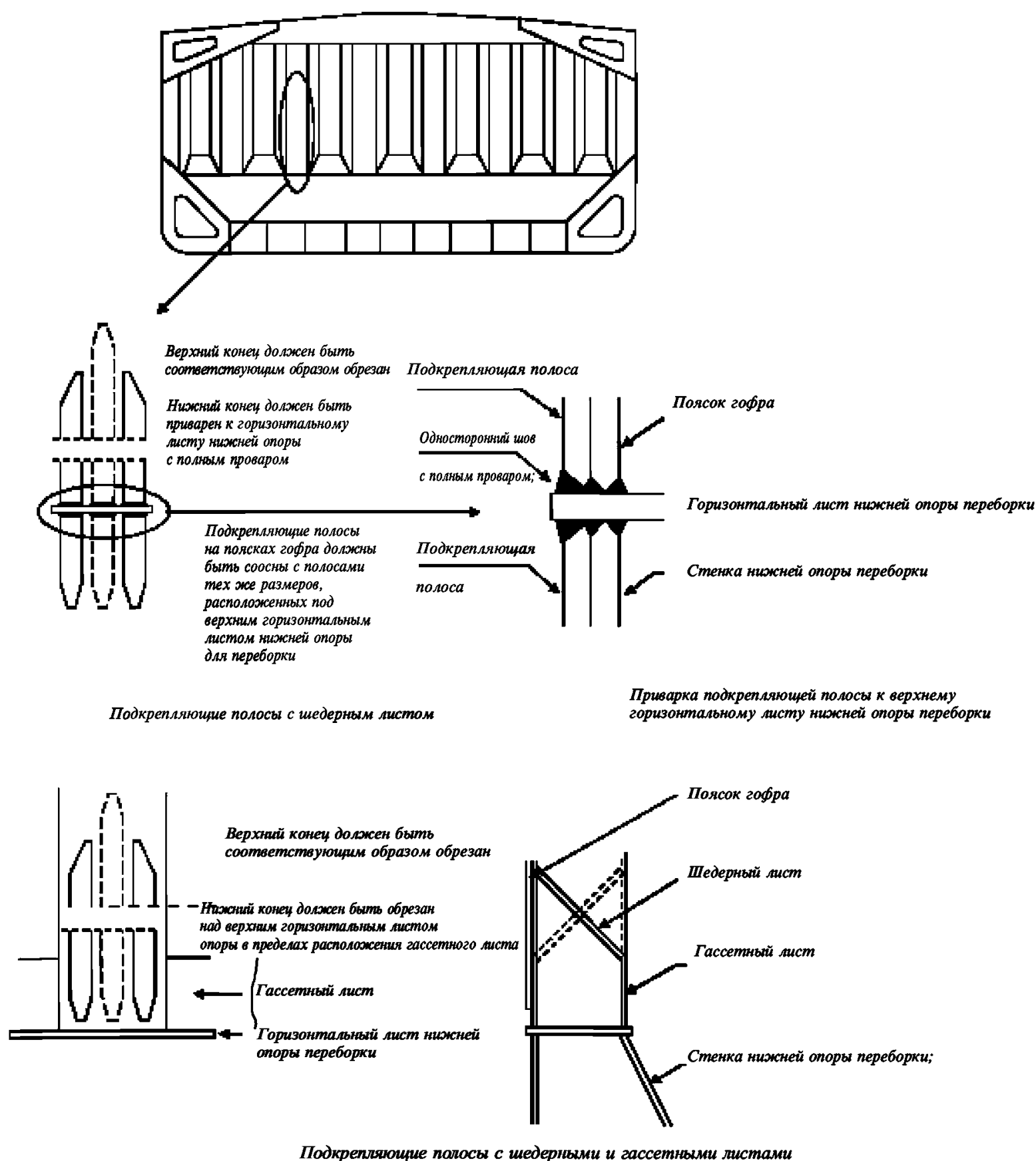
Рис. 1 Общая схема подкрепления переборки.
