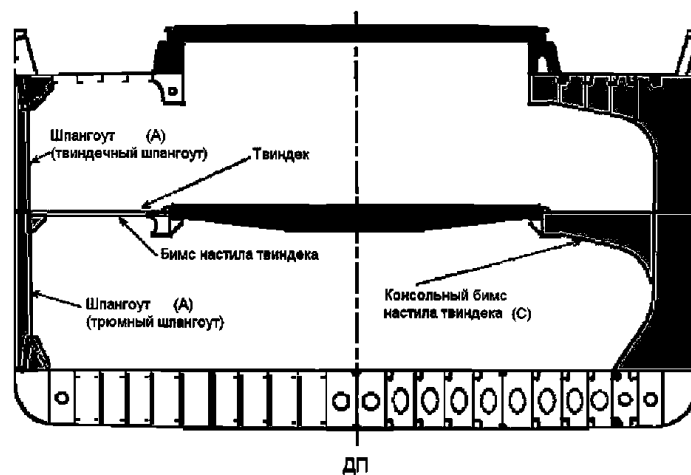
Рис. 7.2.3.2-2 Районы А, С, D и F детального освидетельствования судов, предназначенных для перевозки сухих генеральных грузов
