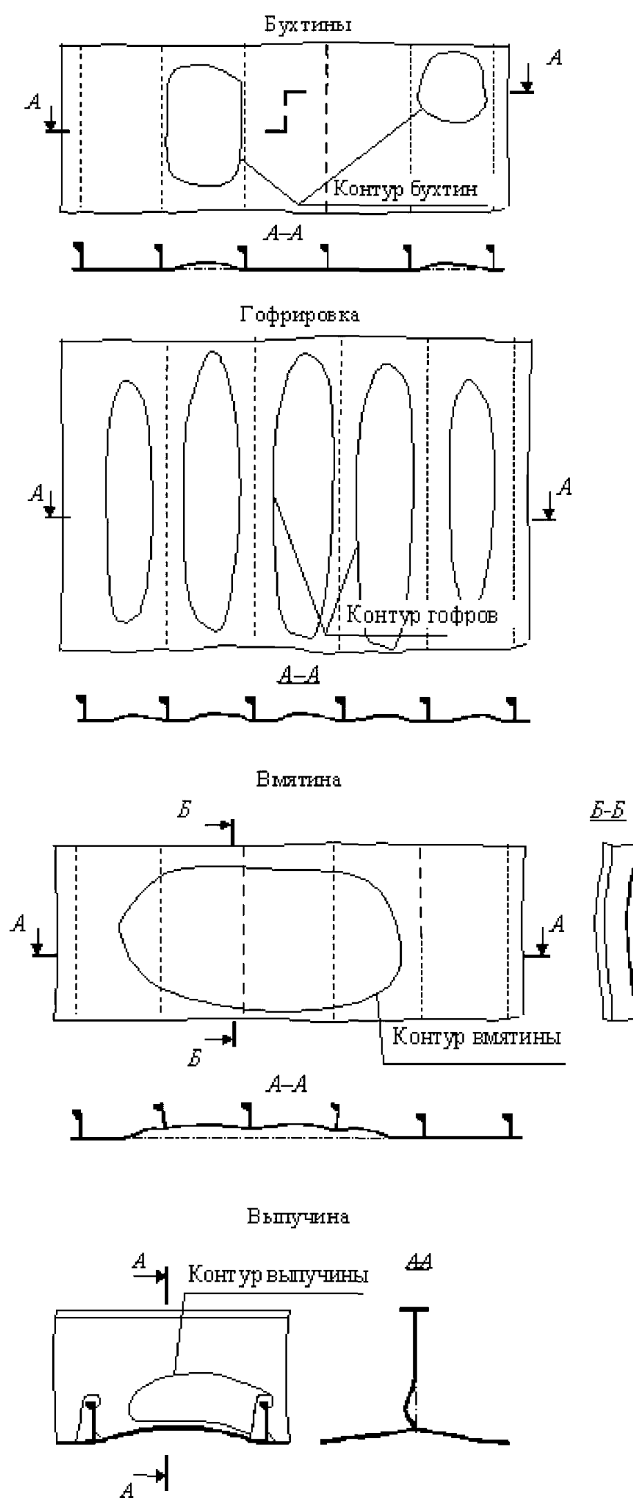
Рис. 1.2.1-1 Виды остаточных деформаций
