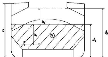
Рис. 5.9.2.2 Схема загруженного трюма ( V — объем груза \text{м}^3 ; P — расчетная точка)
