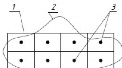
Рисунок Г.1 — Пример расположения контрольных точек для измерения горизонтальной освещенности на пешеходных дорожках и аллеях
