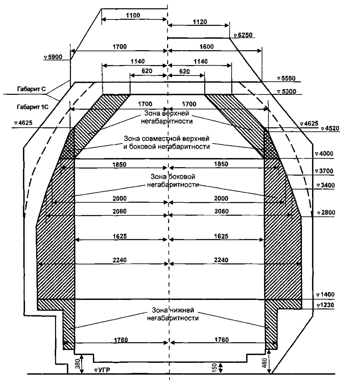
Рис.1. Зоны негабаритности груза
