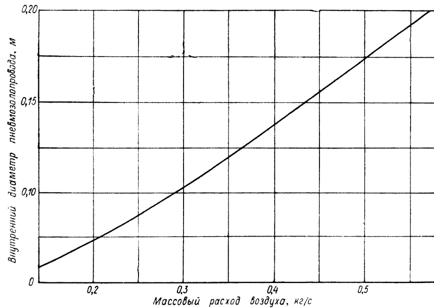
Рис. 4. Зависимость диаметра пневмошлангопровода от массового расхода воздуха.
