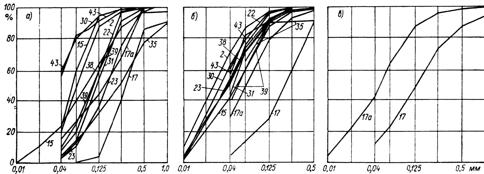
Рис. 15. Кривые гранулометрического состава инерционных золоуловителей (группа 2)
