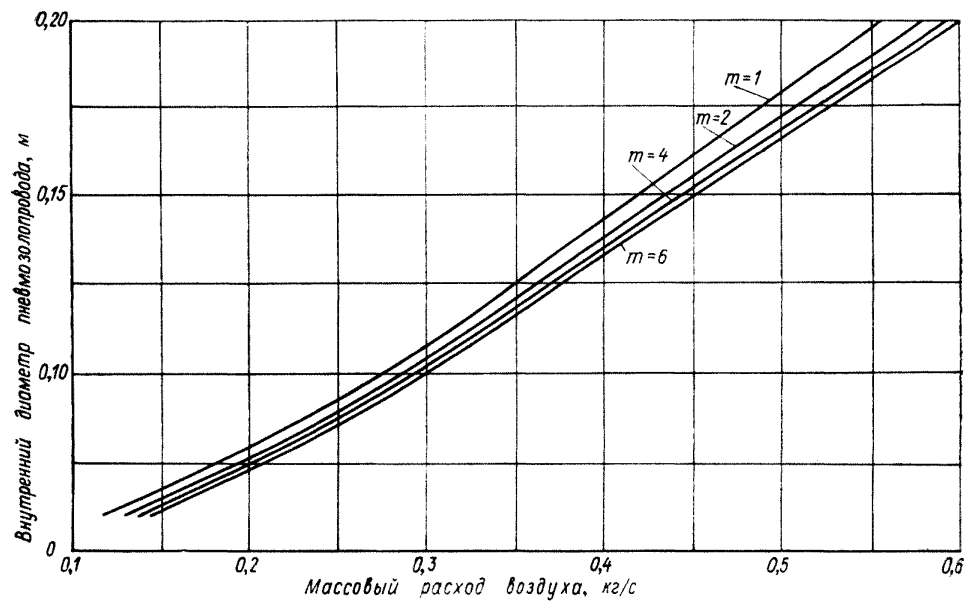
Рис. 3. Зависимость диаметра пневмоизопровода от массового расхода воздуха.
