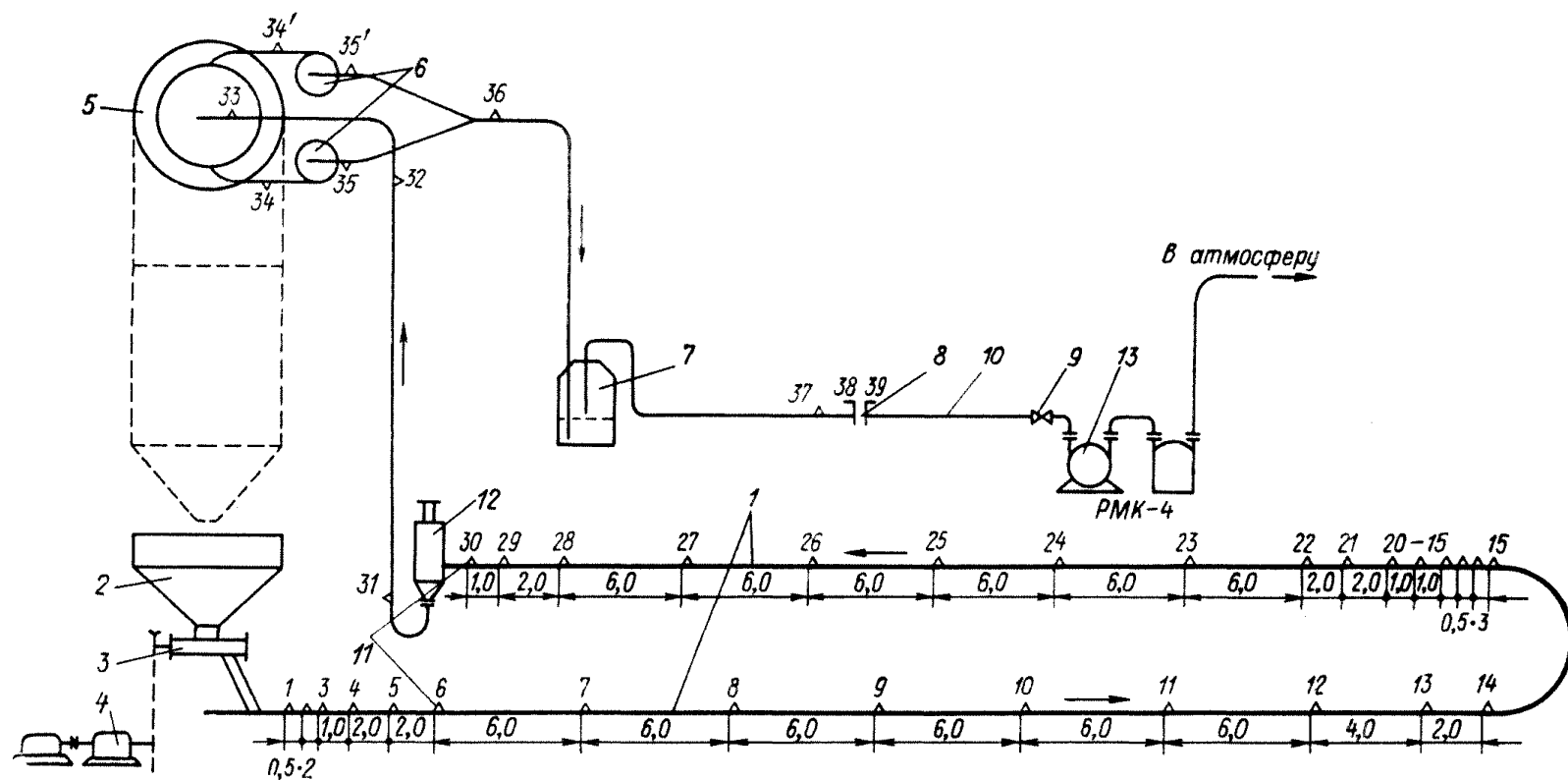
Рис. 18. Схема вакуумной пневмотранспортной установки
