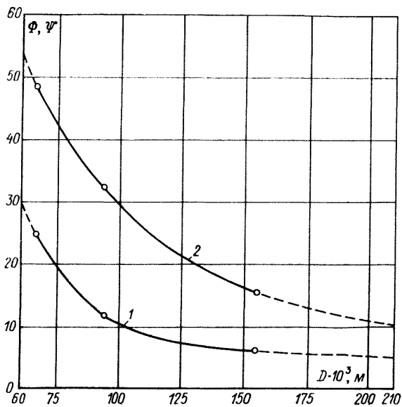
Рис. 21. Опытные корректирующие функции для определения критических скоростей 1 - \varphi = f(D \cdot 10^3) ; 2 - \psi = f(D \cdot 10^3) .
