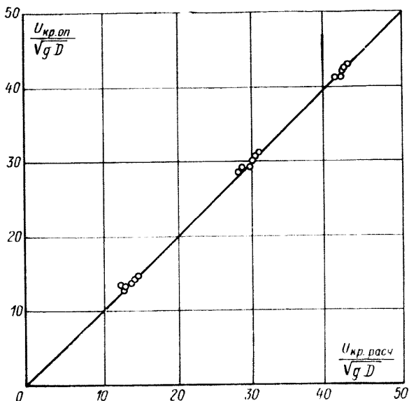
Рис. 22. Сравнение опытных и расчетных значений критических скоростей.
