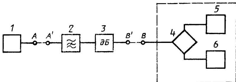
1 — источник входного сигнала; 2 — режекторный фильтр; 3 — аттенюатор; 4 — дуплексер испытуемой аппаратуры; 5 — передающая часть аппаратуры; 6 — приемная часть аппаратуры
