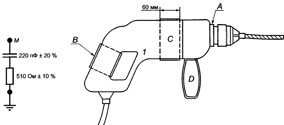
Рисунок 8a) — Элемент RC
