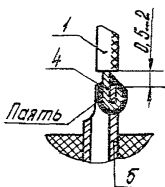
в) запайка сверху
