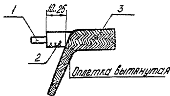
I - жила провода; 2 - изоляция провода; 3 - экранирующая оплетка
