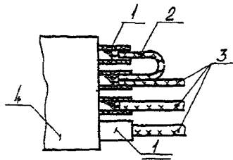
1 - трубка изоляционная; 2 - перемычка; 3 - провода; 4 - корпус соединителя
