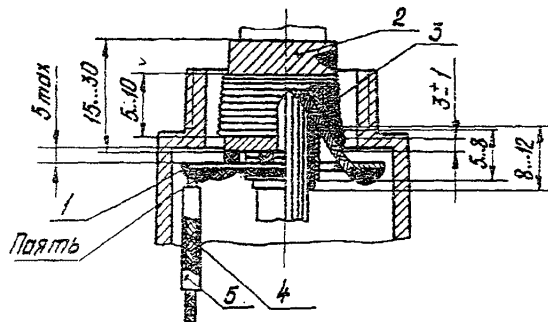
I - шайба; 2 - лента изоляционная; 3 - биндаж нитяной; 4 - плетенка заземления; 5 - трубка изоляционная
