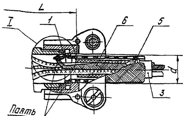
б) Экранированная заделка
