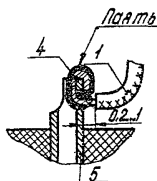
г) запайка сбоку
