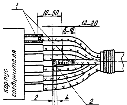
1 - трубка изоляционная; 2 - бандаж нитяной
