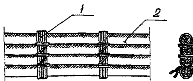
I - биндаж нитяной; 2 - кабель плоский
