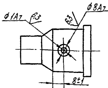
2. Прямые фланцевые патрубки соединителей серии ШР, Р, СШР и 2РТ Для соединителей серии ШР до 10 контактов диаметр отверстия сверления диаметром 4 мм на расстоянии 4 мм.
