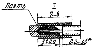
а) контакт соединителя РС
