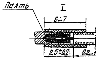
б) контакт соединителя МР
