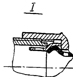
Заделка наружного экрана
