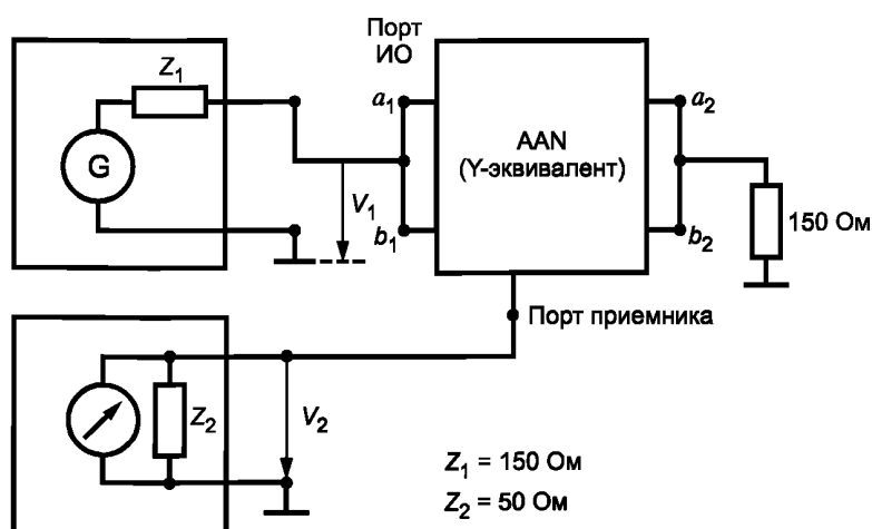
Рисунок Е.8 — Испытательная установка для калибровки коэффициента деления напряжения ААН, дБ, для асимметричной схемы:
