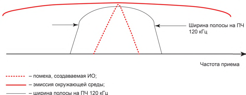
Рисунок A.8 — Немодулированная помеха от ИО (точечная кривая)
