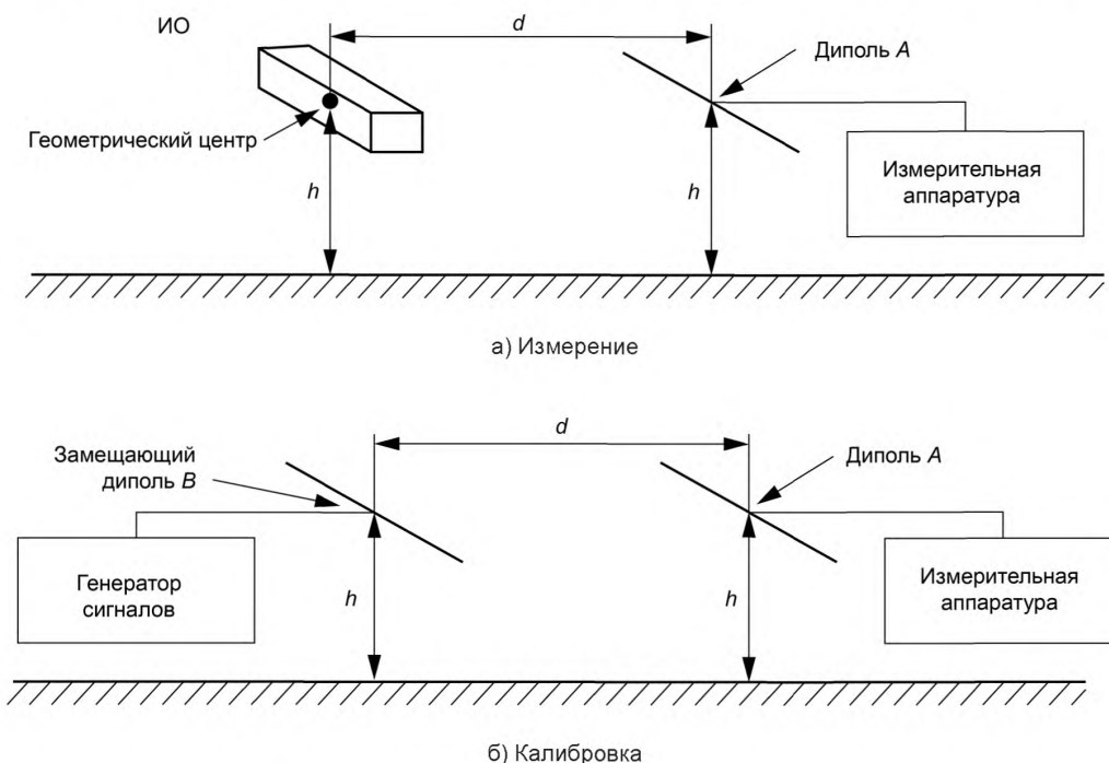
Рисунок 18 — Геометрия испытательной установки при методе замещения
