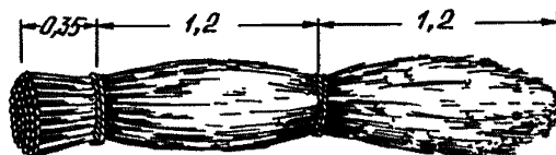
Рис. 14. Однокомельная фашина
