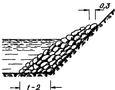
Рис. 1. Каменная наброска (средняя толщина наброски 0,65—1 м)
