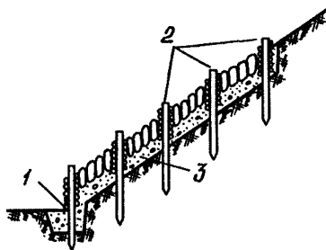
Рис. 4. Мощение в плетневых клетках: 1 — плетневая заборка; 2 — плетень; 3 — слой щебня
