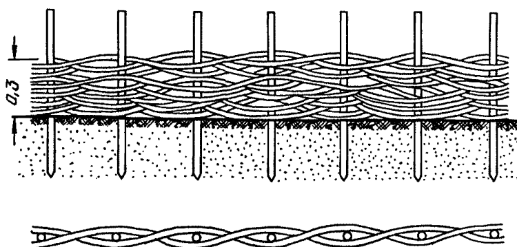
Рис. 8. Плетневая стенка
