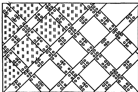
Рис. 7. Одерновка в клетку
