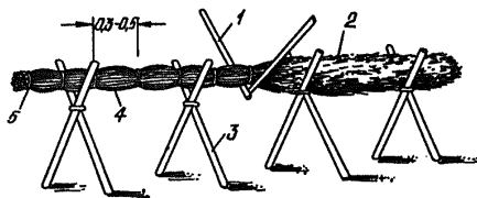
Рис. 12. Вязка хворостяного каната: 1 — сжим; 2 — хворост; 3 — козлы; 4 — канат; 5 — перевязка
