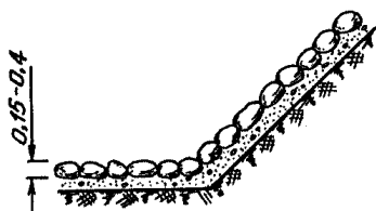
Рис. 3. Мощение камнем
