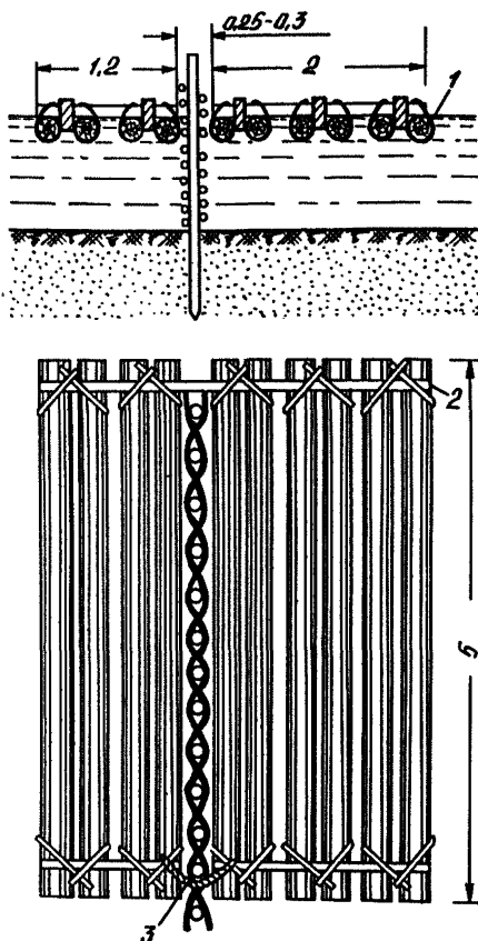
Рис. 10. Плот для устройства плотня: 1 — неокоренные еловые бревна диаметром 0,2; 2 — жердь диаметром 0,1; 3 — чалка диаметром 0,02
