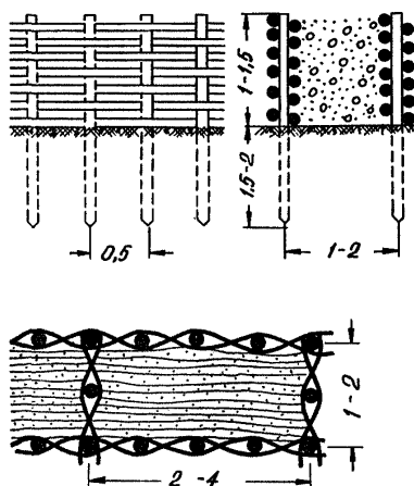
Рис. 11. Двухрядный плетень
