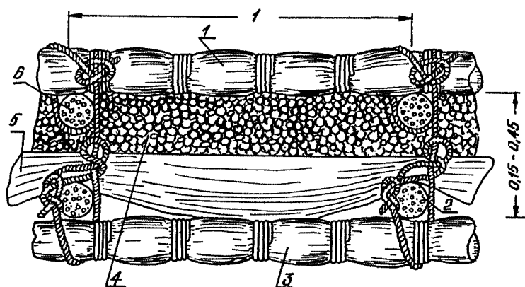
Рис. 9. Хворостяной тюфяк (разрез): 1 — верхний канат верхней сетки; 2 — верхний канат нижней сетки; 3 — нижний канат нижней сетки; 4 — верхний слой хвороста; 5 — нижний слой хвороста; 6 — нижний канат верхней сетки
