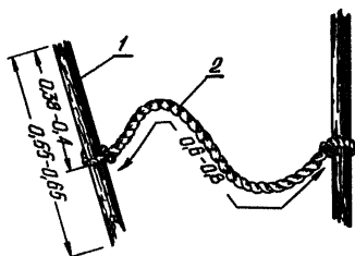
Рис. 13. Веревоочный сжим: 1 — палка; 2 — веревка
