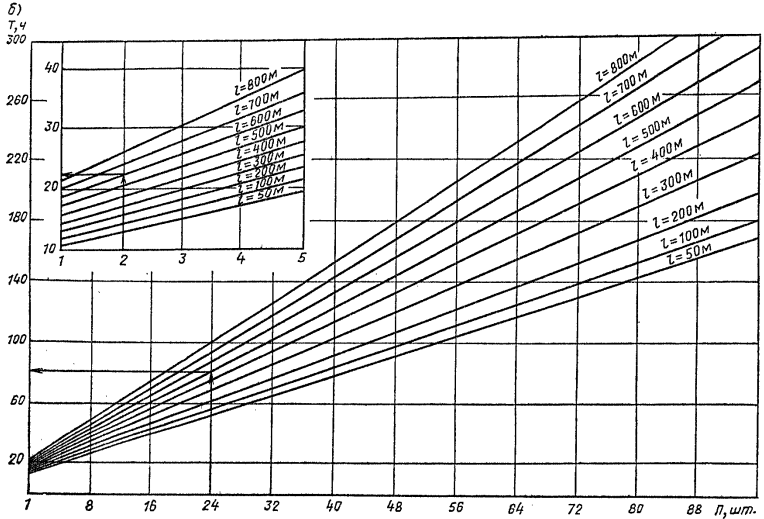
Рис. 2. Номограммы для определения продолжительности ТО T дренажных установок водяного (а) и пенного (б) пожаротушения в зависимости от количества направлений (контрольно-пусковых узлов) П
