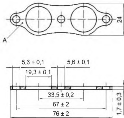
Рисунок 4 – Пластика для удерживания колец
