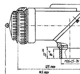
Розетка кабельная с угловым кожухом и замком
