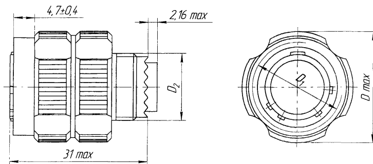
Вилка (розетка) кабельная
