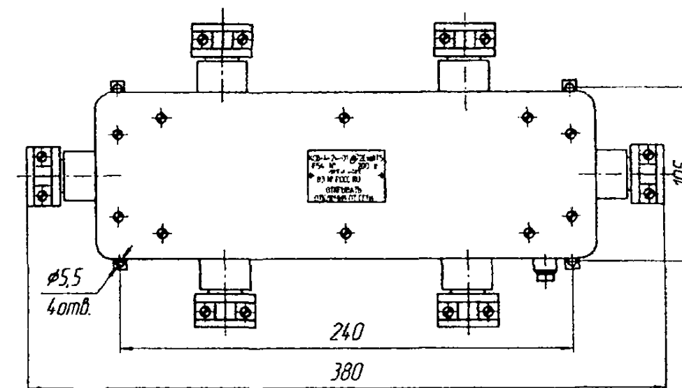
КСВ-4-24-01, КСВ-4-24-02, КСВ-4-24-03, КСВ-4-24-04, КСВ-4-24-05, КСВ-4-24-14
