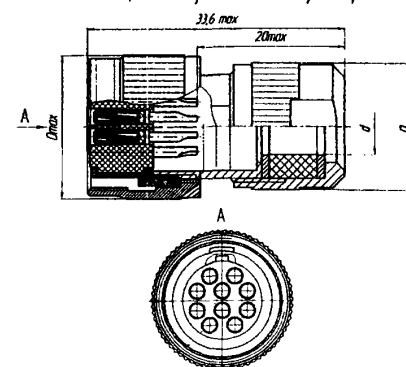
Розетка УЗНЦ05 с прямым незэкранированным кожухом
