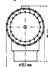
Розетка кабельная с угловым кожухом и замком
