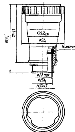
Вилка (розетка) 9Р1С(Т)-102А(В)
