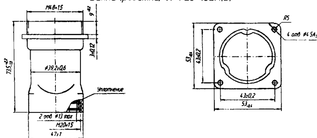
Вилка (розетка) 9РФ23-102А(В)
