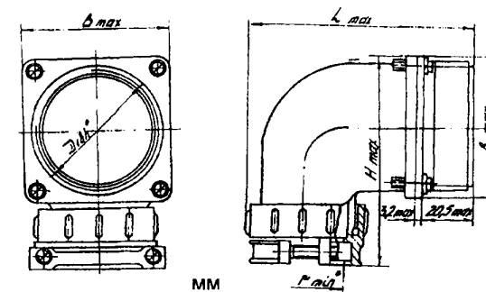
Вилки (розетки) с угловым патрубком и гайкой для неэкранированного кабеля
