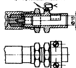
Рис.1. Габаритные, установочные и присоединительные размеры коробок типа 1.
