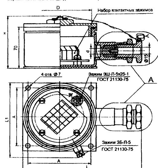
Рис.1. Габаритные, установочные и присоединительные размеры коробок типа 1.
