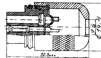
Вилки РВН2-7, РВН3-7
