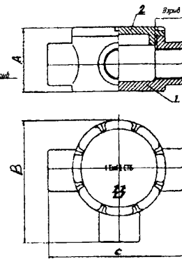
Коробка тройниковая алюминиевая типа КТА-20, КТА-25. 1- корпус, 2- крышка Рисунок 2.
