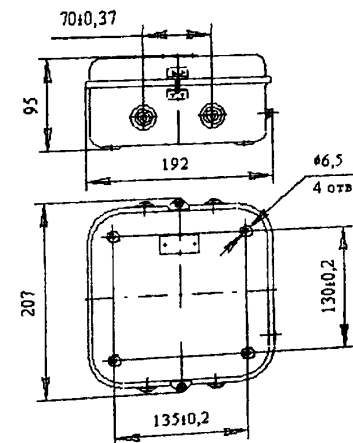
БЗК-40.16, БЗК-40.25 и БЗК-40.32
