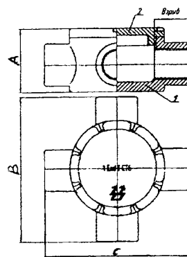
Коробка крестовая алюминиевая типа ККА-20, ККА-25. 1- корпус, 2- крышка Рисунок 1.
