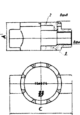
Коробка проходная алюминиевая типа КПА-20, КПА-25. 1- корпус, 2- крышка Рисунок 3.
