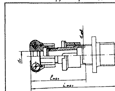
Патрубки прямые для неэкранированного кабеля (ПН)
