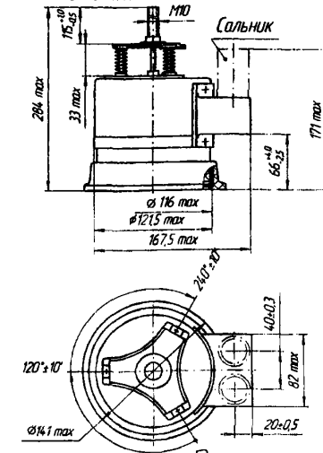
Розетка РА-153 3.645.145Сп
