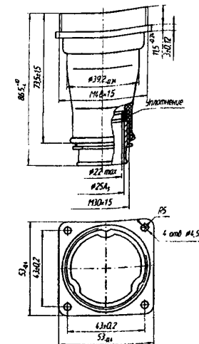
Вилка (розетка) 9РФ1С-102А(В)
