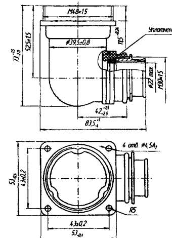
Вилка (розетка) 9РФУ1С-102А(В)
