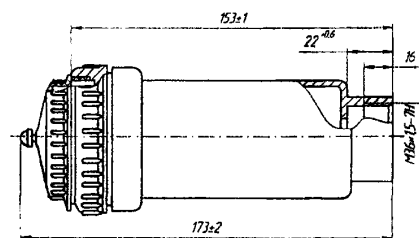
Розетка кабельная с прямым кожухом и замком
