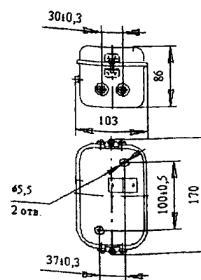
Габаритные и установочные размеры блоков
