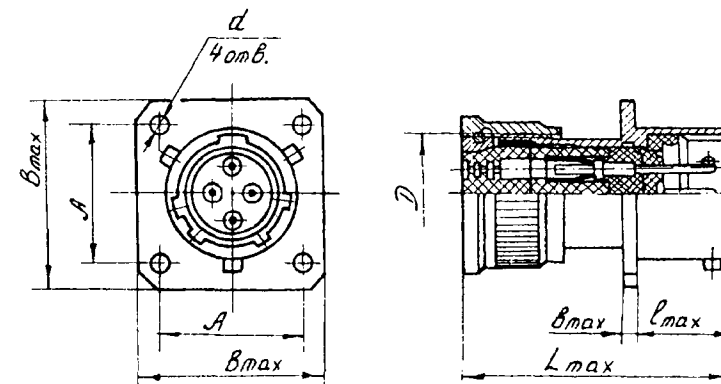
Соединители СНЦ23 приборные
