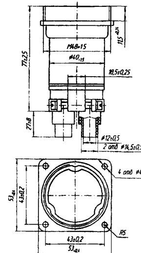
Вилка (розетка) 9РФ2С-102А(В)
