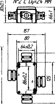
КП 6 для вводов №2 с Ø у =24 мм
