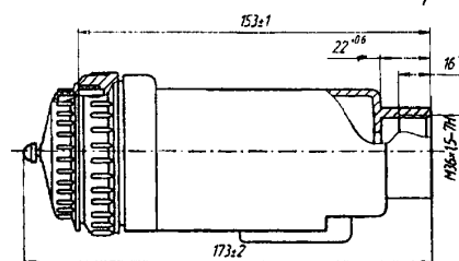
Розетка кабельная с угловым кожухом
