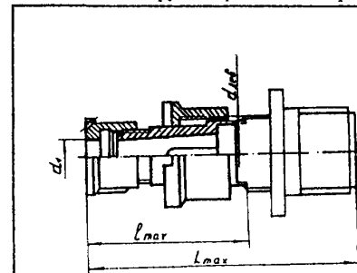
Патрубки прямые для экранированного кабеля (ПЭ).
