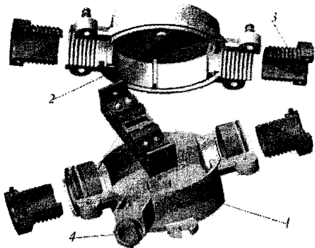
1 – корпус; 2 – крышка; 3 – полное разъемное уплотнительное устройство для магистрального кабеля; 4 – уплотнительный ввод для проводников ответвительной цепи.
