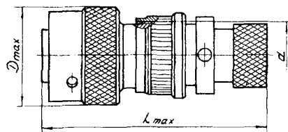
Соединители СНЦ 23 кабельные, с обоймой под термоусаживающиеся трубки
