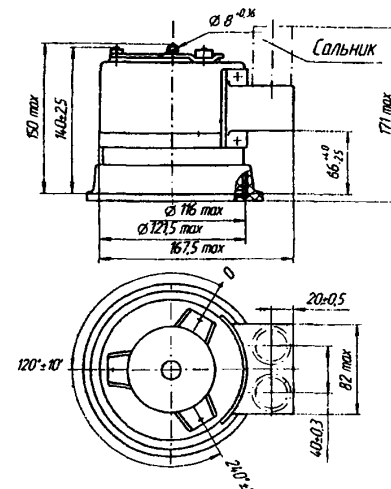
Розетка РА-153 3.645.145Сп
