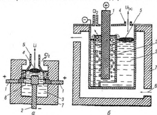
а – диафрагменный электролизер:
