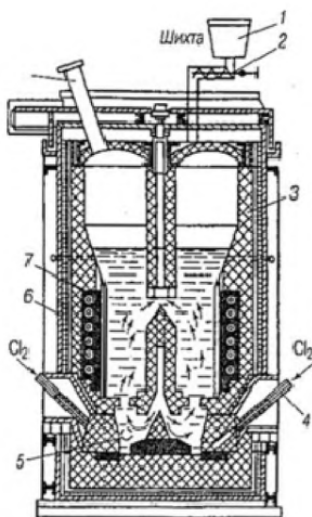
1 – шихтоприемник; 2 – транспортер-дозатор; 3 – шамотная футеровка; 4 – фурма 5 – летка; 6 – корпус; 7 – графитовые нагреватели; 8 – газоход
