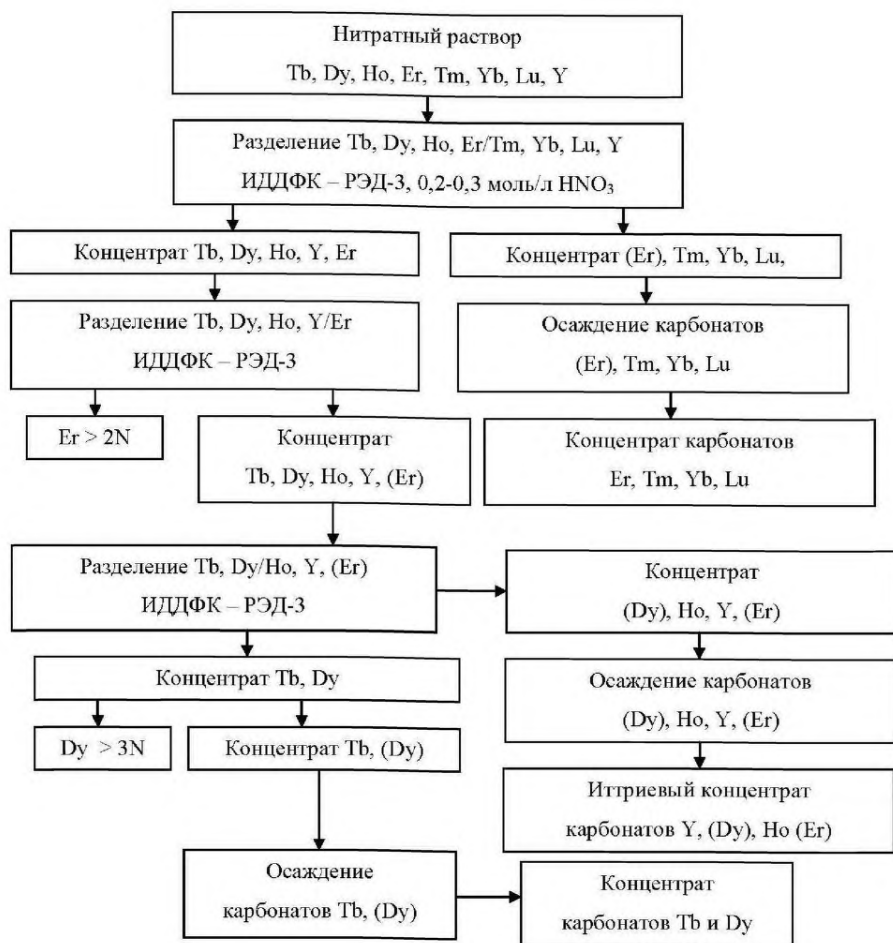
Рисунок 2.29 – Схема разделения иттрий-эрибиевого концентрата, полученного при переработке различного минерального сырья
