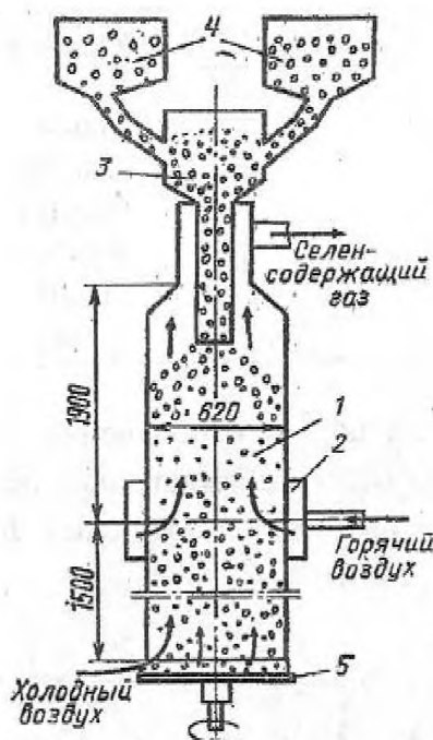
Рисунок 2.5 Шахтная печь окислительного обжига шлама непрерывного действия
