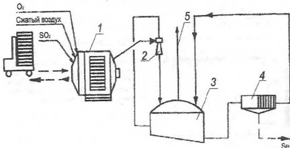
1 – печь обжига селена; 2 – эжектор; 3 – циркуляционная емкость; 4 – фильтр-пресс; 5 – очищенный от диоксида селена газ
