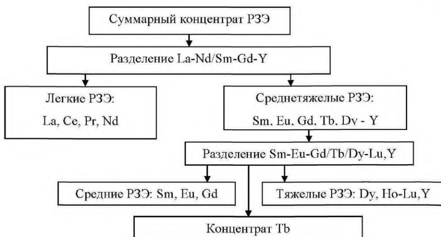
Рисунок 2.15 – Схема 1 разделения группового бастинезитового концентрата РЗЭ, реализованная на предприятиях в Китае
