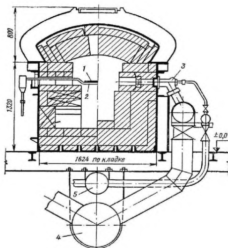
1 – нагреваемый штрипс; 2 – глissажные трубы, охлаждаемые водой; 3 – горелки; 4 – газовый коллектор; 5 – воздушный коллектор
