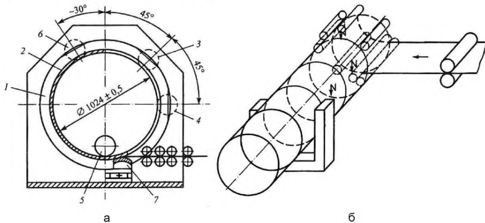
Рисунок 2.46 – Поперечный разрез формовочного стана полувтулочного типа (а) и схема сварки спиральношовных труб под слоем флюса (б)
