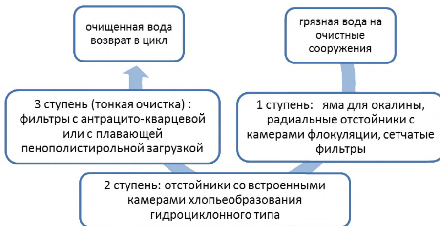
Рисунок 3.3 – Трехступенчатая схема очистки сточных вод станов горячей прокатки
