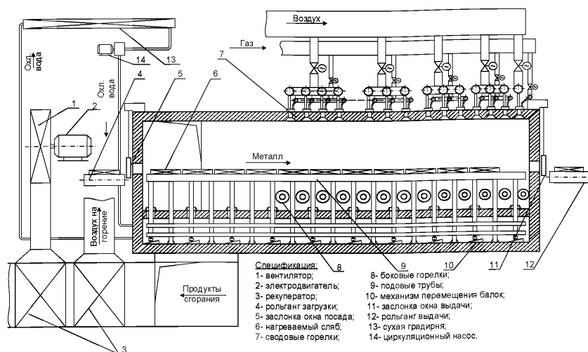
Рисунок 7.8 – Схема нагревательной печи для нагрева слэбов
