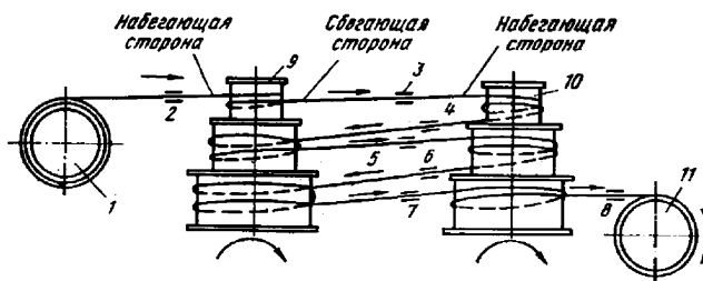
1 – фигурка с проволокой; 2–8 – волокни; 9, 10 – ступенчатые барабаны; 11 – приемный барабан
