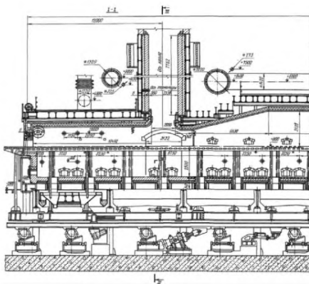
а) продольный разрез
