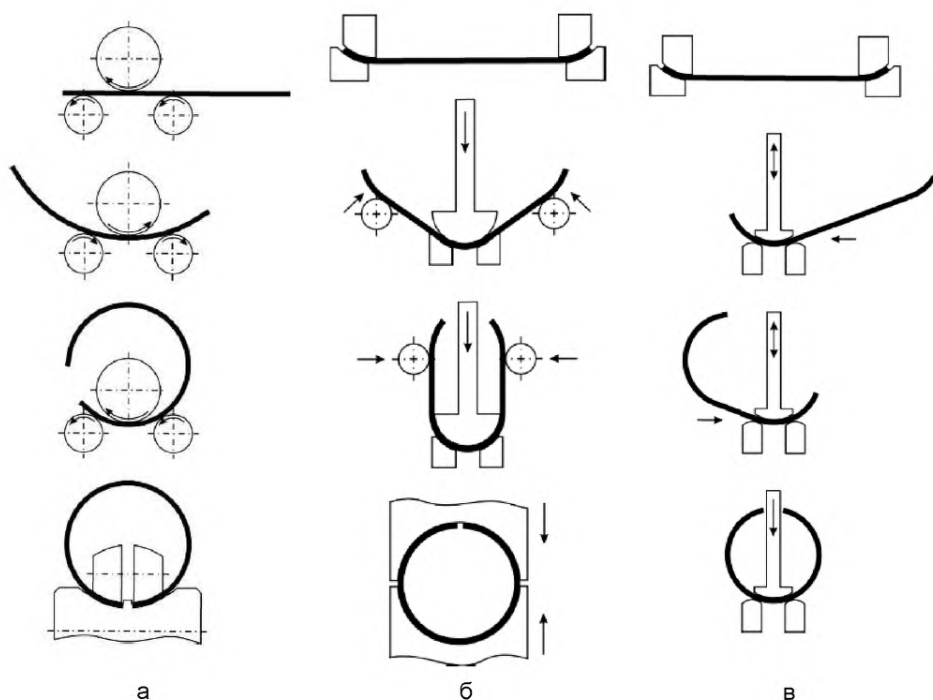
а – в гибочных вальцах; б – на прессе при производстве труб с одним прямым швом (UO-формовка); в – на прессе при производстве труб с одним прямым швом (JCO-формовка)
