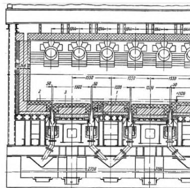
б) поперечный разрез
