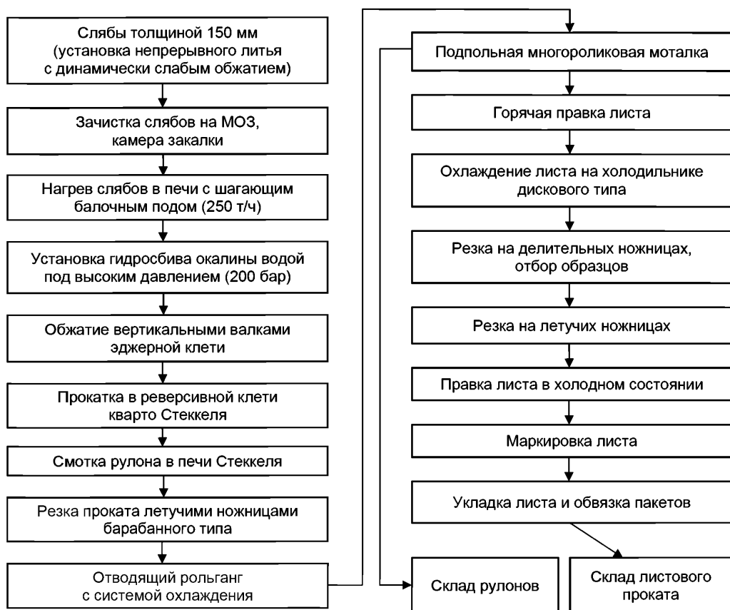
Рисунок 7.3 – Технологическая схема производства непрерывнолитых слэбов и горячекатаного листа
