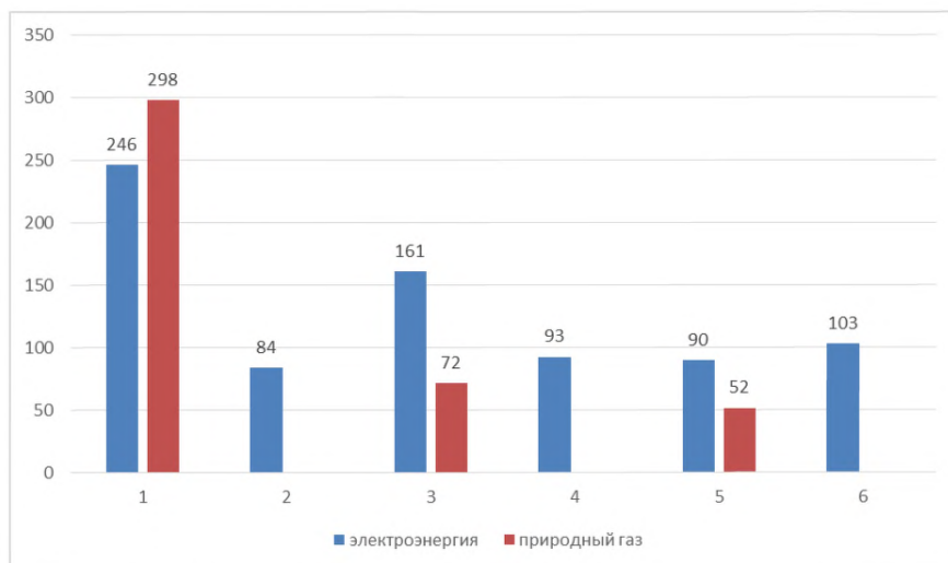
Рисунок 3.4 – Удельное потребление электроэнергии (кВт·ч/т) и природного газа (м³/т) [по данным анкет].
