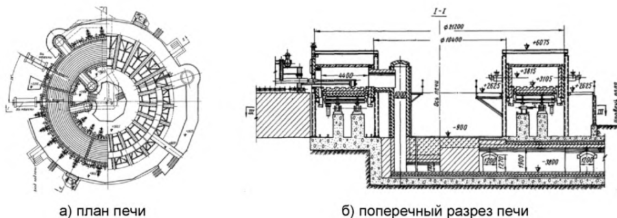
Рисунок 2.20 – Кольцевая печь [30]
