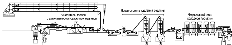
Рисунок 7.4 – Линия бесконечной холодной прокатки полос разработки фирмы INI
