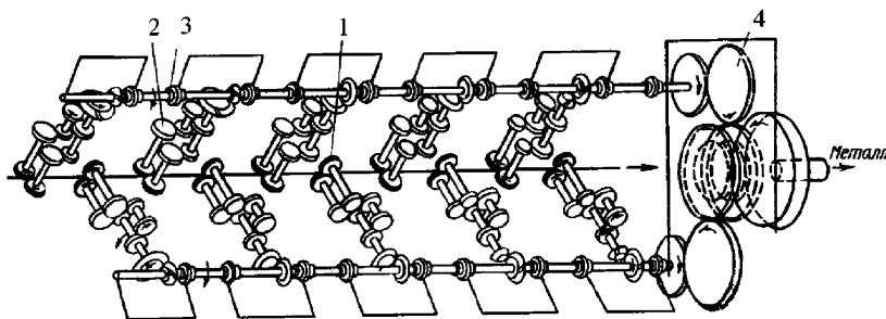
1 – прокатные валки; 2 – шестеренные валки; 3 – трансмиссия; 4 – главный редуктор
