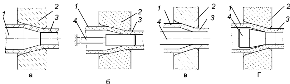
а – безоправки; б – на короткой неподвижной оправке; в – на длинной подвижной оправке; г – на самоустанавливающейся оправке; 1 – исходная заготовка; 2 – волокна; 3 – готовая труба; 4 – оправка
