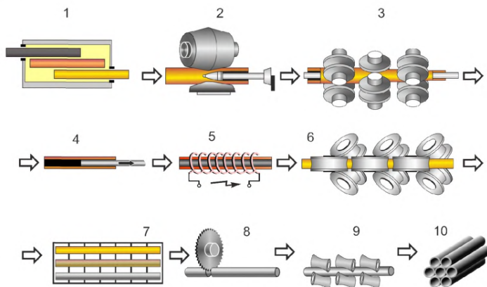
1 – нагрев заготовок; 2 – прошивка заготовок; 3 – прокатка гильз в непрерывном стане; 4 – извлечение оправки; 5 – промежуточный нагрев труб; 6 – калибрование, редуцирование труб; 7 – охлаждение труб; 8 – обрезка концов труб, порезка труб на мерные длины; 9 – правка; 9 – передача труб на промежуточный склад
