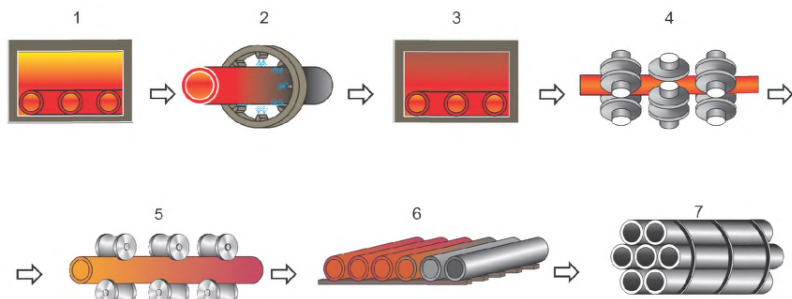
1 – нагрев труб в закалочной печи; 2 – охлаждение труб в закалочном устройстве; 3 – нагрев труб в отпускной печи; 4 – калибрование труб; 5 – правка; 6 – охлаждение труб; 7 – передача труб на промежуточный склад.
