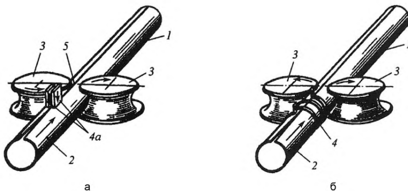
1 – сварная труба; 2 – сформованная заготовка; 3 – сварочные валки; 4 – индуктор; 4а – скользящий контакт; 5 – место сварки
