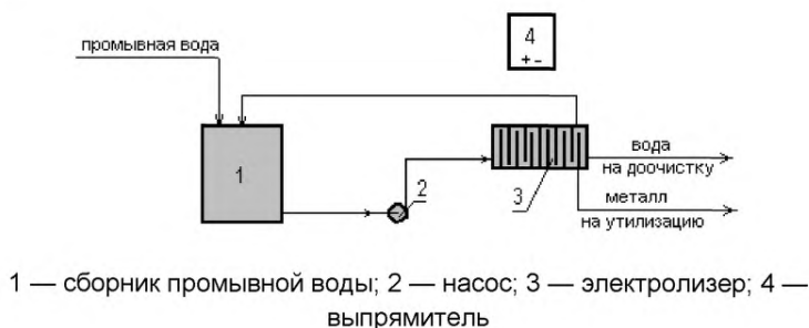
Рисунок 2.27 — Принципиальная схема очистки сточной воды методом электролиза
