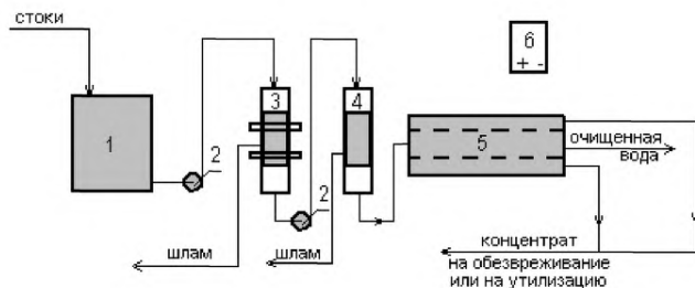
1 — накопитель стоков; 2 — насос; 3 — механический фильтр; 4 — сорбционный фильтр; 5 — электродиализатор; 6 — выпрямитель
