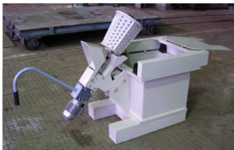
Рисунок 2.12 — Общий вид колокольной ванны погружного типа
