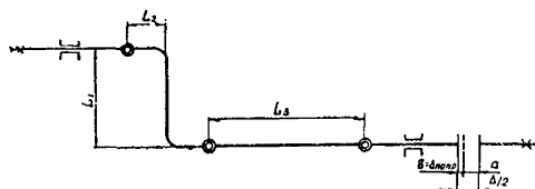
КБУ: в) Z-образная шарнирная система с тремя компенсаторами КБУ.
