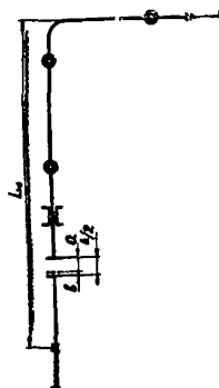
КБУ: а) угловая шарнирная система для обслуживания одного трубного пролета (компенсаторы КБУ).
