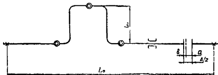
КБУ: д) П-образная шарнирная система.
