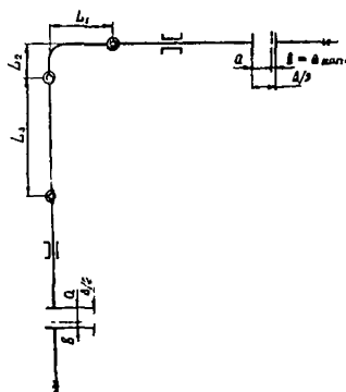
КБУ: б) угловая шарнирная система для обслуживания двух трубных пролетов (компенсаторы КБУ).
