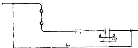
КБУ: г) Z-образная шарнирная система с применением двух компенсаторов КБУ.
