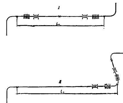
КВО: I — на прямом участке; II — на повороте.
