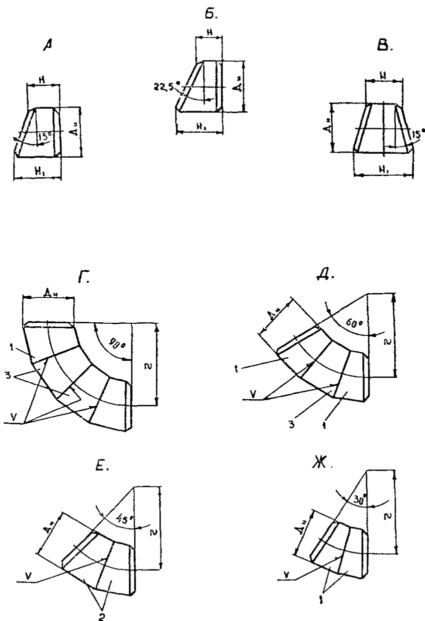
Рис. 1-П. Отводы сварные из углеродистой и легированной сталей на R_y до 64 кгс/см 2 :
