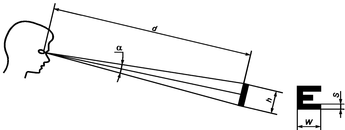
d — расстояние между глазом и знаком; α — угол зрения знака . . . °; h — высота знака; w — ширина знака; s — толщина линий знака
