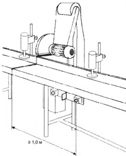
Рисунок 2 – Расположение двухручного органа управления на полуавтоматических станках
