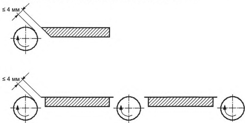
Рисунок 6 – Пример защиты роликового конвейера
