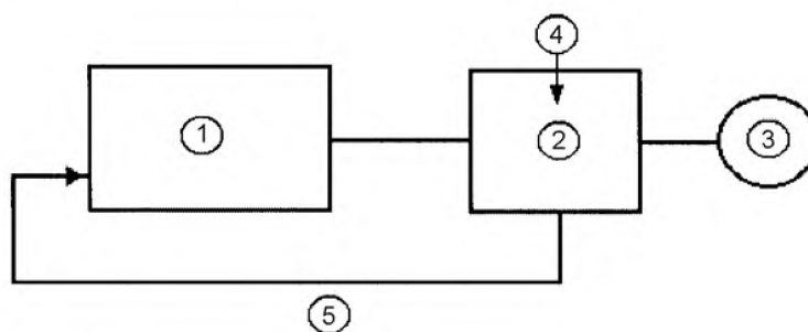
Рисунок А.3 – Система управления, связанная с безопасностью, для включения двигателя пилы
