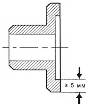
Рисунок 3 – Фланец пилы
