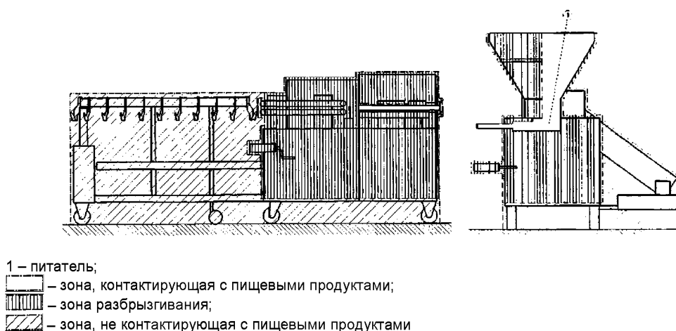
Рисунок 28 – Гигиенические зоны машин с цилиндром и загрузочным питающим бункером
