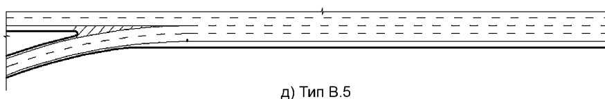
Рисунок В.1 — Основные схемы организации участков примыкания транспортных потоков
