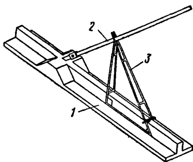
Рис. 5. Плита с прикрепленной анкерной тягой
