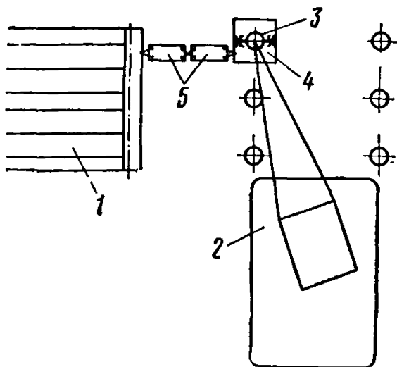
Рис. 11. Установка железобетонных днищ в полости колонн-оболочек
