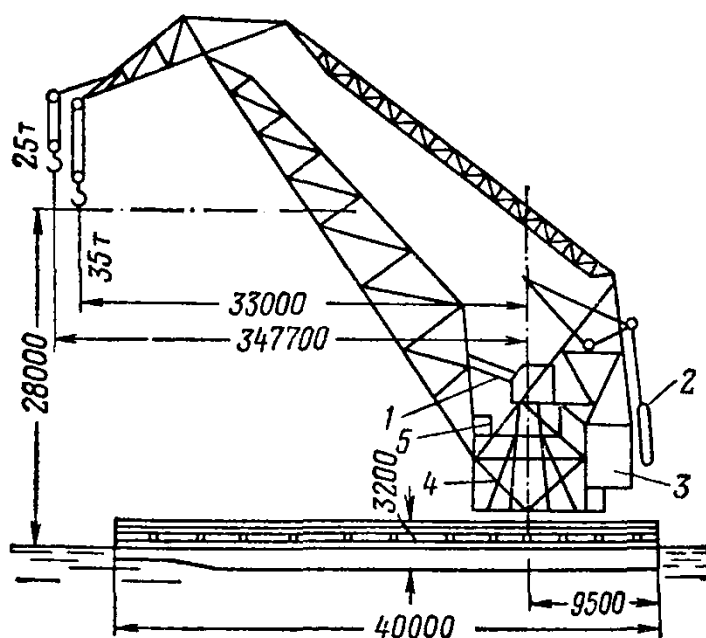
Рис. 29. Схема плавучего 100-т крана «Ганц».
