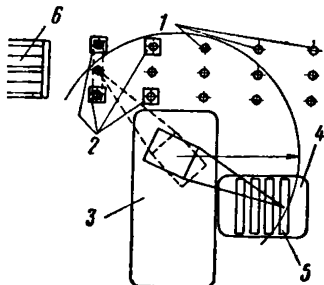
Рис. 12. Схема установки ригелей на свайные ряды из колонн-оболочек
