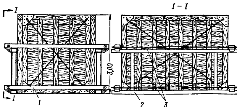
Рис. 22. Деревометаллическая опалубка обыкновенных массивов 1 — металлическая балка; 2 — металлическая плоская рама; 3 — стяжки
