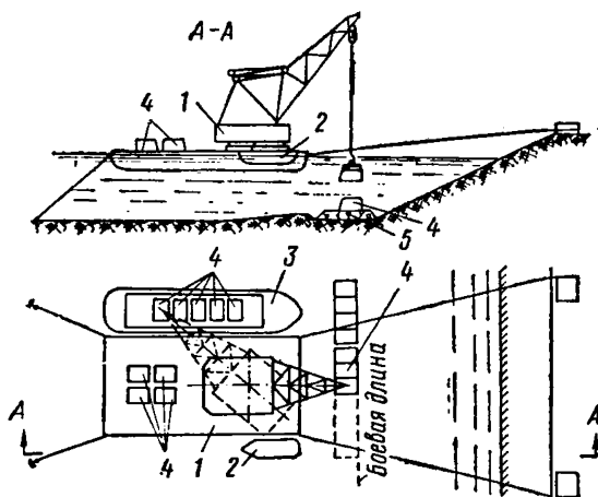
Рис. 3. Схема монтажа стенки из правильной массивовой кладки
