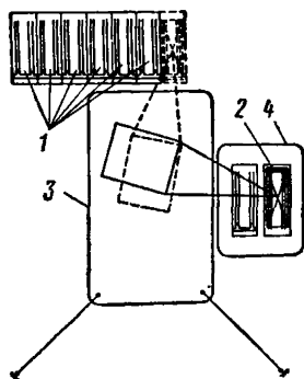
Рис. 7. Схема монтажа причальной набережной из уголковых блоков с внутренним анкером
