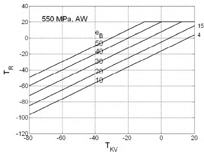
Рисунок В.2-10 – МЕТОД 2. Расчетная номинальная температура и температура испытаний на удар для аустенитно-ферритных сталей, e_B \leq 50 мм, R_e = 465 МПа и KV \geq 40 Дж
