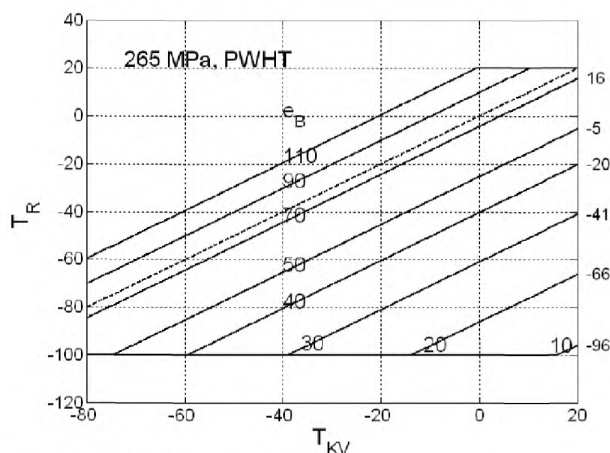
Рисунок В.2-1 – МЕТОД 2. Расчетная номинальная температура и температура испытаний на удар в состоянии термической обработки после сварки (PWHT) для R_e \leq 265 МПа и KV \geq 27 Дж. Пунктирная линия используется только для KV \geq 40 Дж и для толщины от 75 до 110 мм включительно
