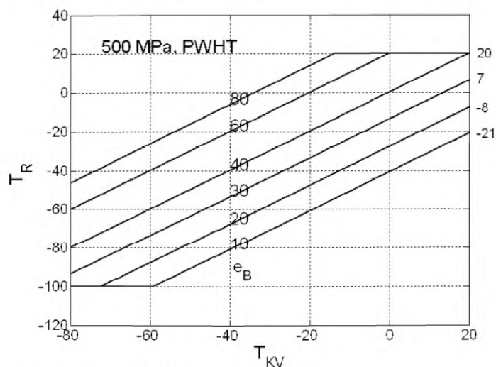
Рисунок В.2-6 – МЕТОД 2. Расчетная номинальная температура и температура испытаний на удар в состоянии непосредственно после сварки (AW), R_e \leq 460 МПа и KV \geq 40 Дж
