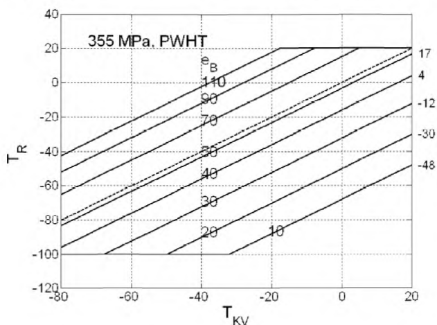
Рисунок В.2-2 – МЕТОД 2. Расчетная номинальная температура и температура испытаний на удар в состоянии непосредственно после сварки (AW) для R_s \leq 265 МПа и KV \geq 27 Дж
