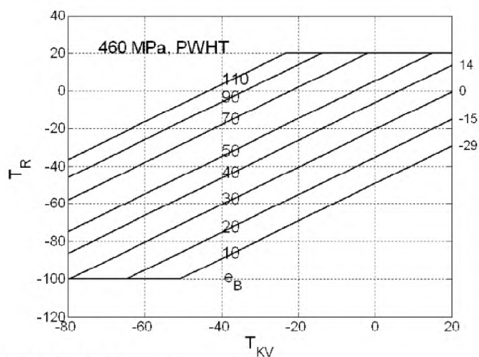
Рисунок В.2-4 – МЕТОД 2. Расчетная номинальная температура и температура испытаний на удар в состоянии непосредственно после сварки (AW), R_s \leq 355 МПа и KV \geq 27 Дж
