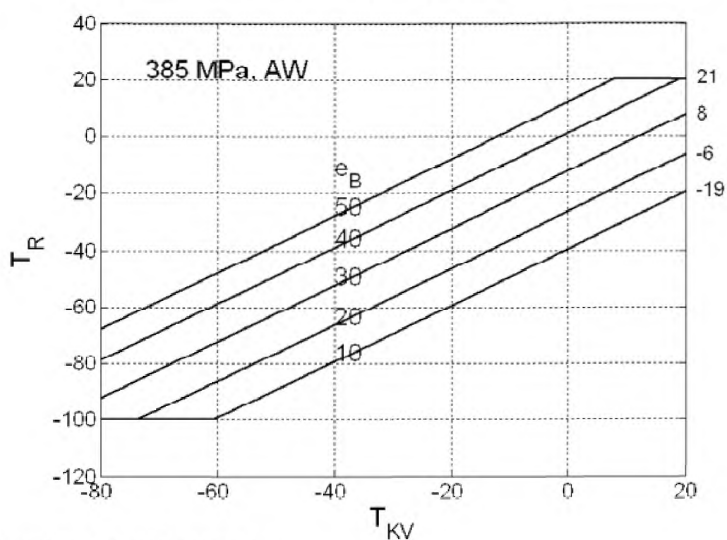
Рисунок В.2-8 – МЕТОД 2. Расчетная номинальная температура и температура испытаний на удар в состоянии непосредственно после сварки (AW), R_e \leq 500 МПа и KV \geq 40 Дж
