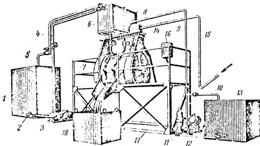
Рис. 3. Принципиальная схема пастосмесительной установки 1—битумный котел; 2, 4, 5—циркуляционный битумопровод от битумоплавильни; 3—битумный насос; 6—дозатор битума; 7—мешалка-пастосмеситель; 8—дозатор суспензии эмульгатора; 9, 10, 12—растворопроводы или резиновые шланги; 11—растворонасос; 13—бункер для эмульгатора; 14—дозатор воды; 15—водопровод горячей воды от котельной; 16—электропитание управления; 17—помост для оператора; 18—емкость для готовой пасты.
