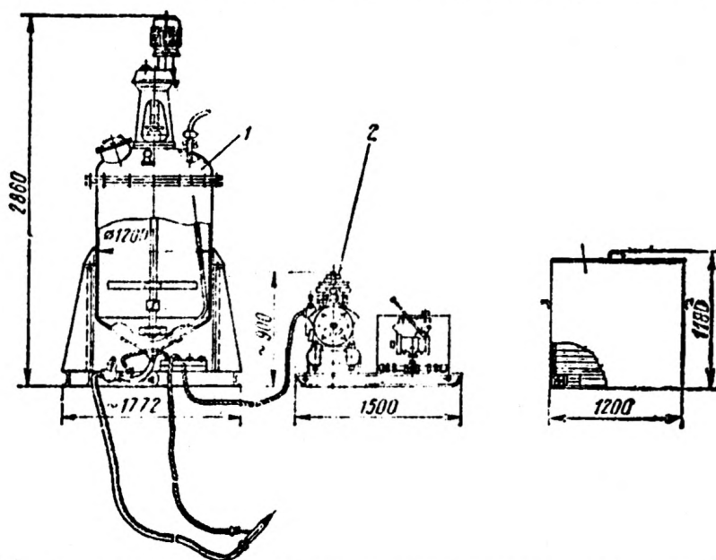
Рис. 10. Установка МД-196 для нанесения холодной асфальтовой гидроизоляции
