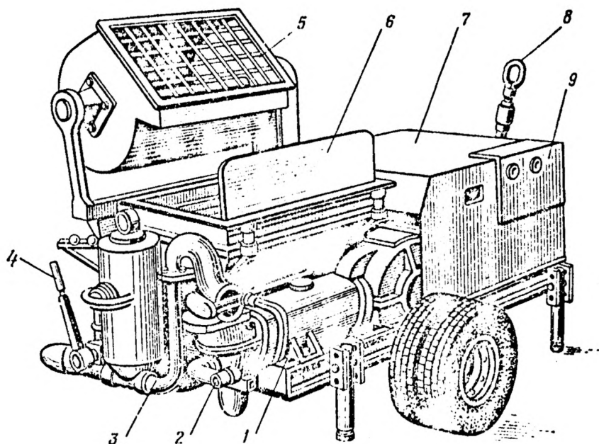
Рис. 9. Растворомесительный агрегат С-372
