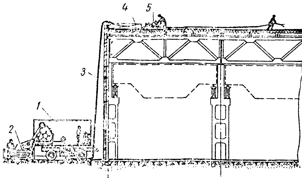
Рис. 14. Технологическая схема организации кровельных работ 1 — смесительно-штукатурная станция ЦННЛ-3; 2 — емкости с пастой и наполнителем; 3 — материалный шланг; 4 — раздаточный бункер на крыше; 5 — дополнительный растворонасос.
