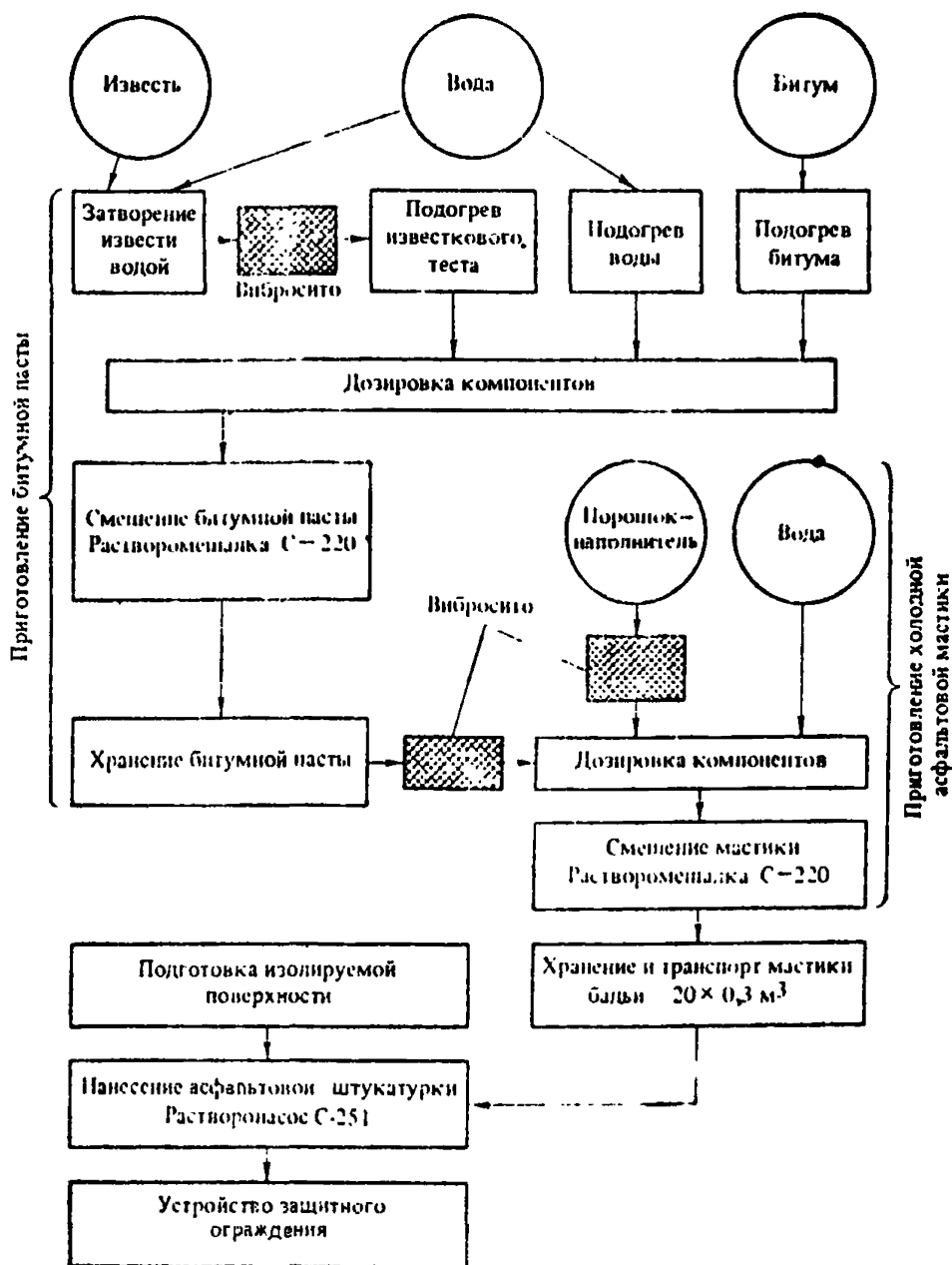
Рис. 2. Технологическая схема устройства холодной асфальтовой гидроизоляции из мастики Хамаег.
