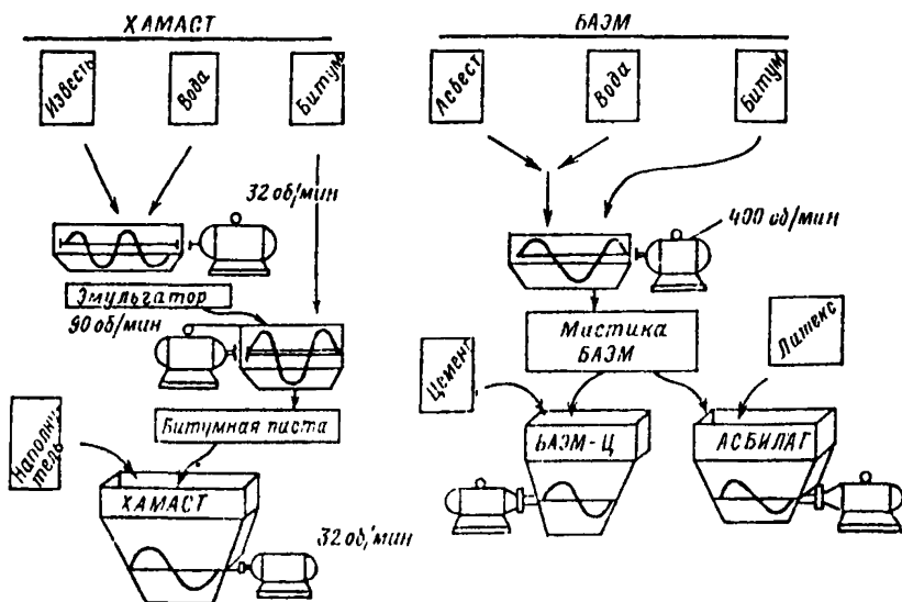
Рис. 1. Технологические схемы приготовления холодных асфальтовых мастик.
