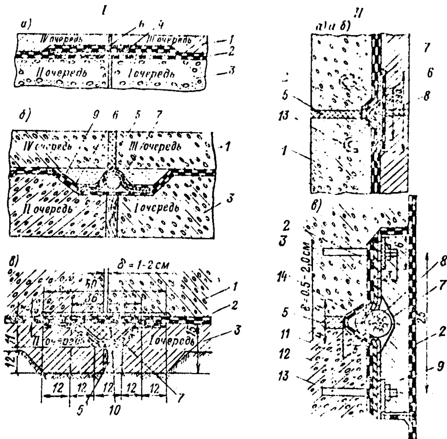
Рис. 7. Сопряжения гидроизоляции с уплотнениями деформационных швов
