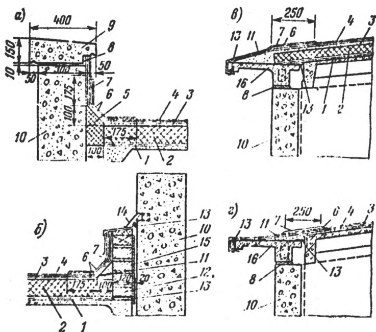
Рис. 13. Сопряжения мастичных кровельных покрытий в случае совмещенных утепленных крыш
