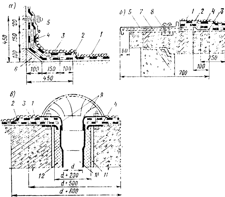
а — с паранетом или стеной; б — с наружным водостокон со свесом; в — с внутренним водостокон — с воронкой; 1 — бронированная накладка; 2 — кровельное покрытие; 3 — дощатый настил; 4 — армирующая стеклоткань; 5 — лист кровельной стали; 6 — плитус из цементного раствора; 7 — антисептированная рейка; 8 — стальной косяк; 9 — зажимной фланец; 10 — чугунная труба; 11 — асбестомеханитная труба; 12 — теплоизоляция.
