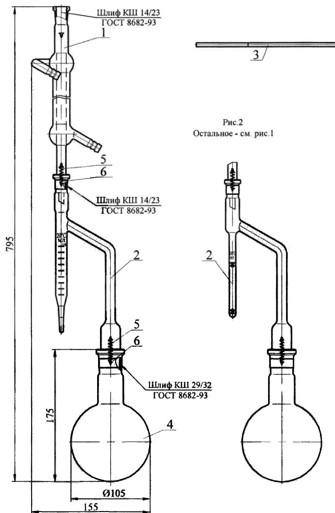
1 - холодильник; 2 - приемник-ловушка; 3 - трубка для распыления; 4 - колба; 5 - пружины; 6 - хомуты
