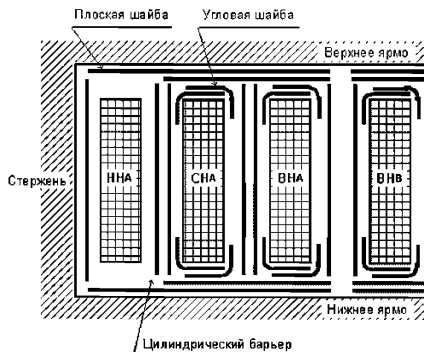
Рисунок А1 – Общий вид главной изоляции обмоток трансформаторов
