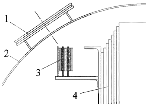
Рисунок 1– Эскиз расположения макета изоляции в баке колокольного типа:
