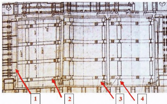
Рисунок 9 – Эскиз конструкции с облегающими обмотки ВН барьерами, барьерами на боковых ямах и зоны отбора образцов
