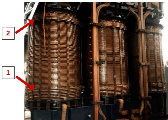
Рисунок 2 – Пример конструкции с вводом линейного напряжения с верхнего и нижнего торца обмотки ВН
