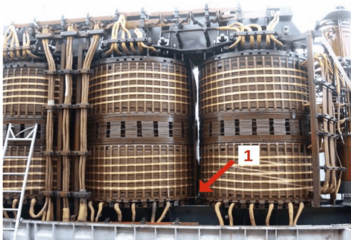
Рисунок 10 – Пример конструкции с наружной РО класса 35 кВ
