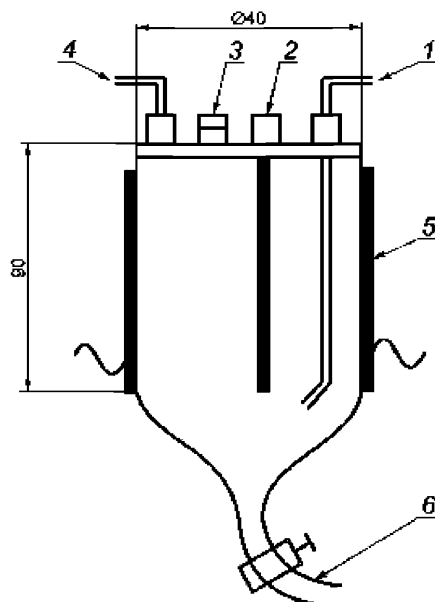
Рисунок В-5 – Стеклоный сосуд испарителя с нагревателем
