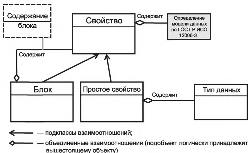
Рисунок 5 — Простые свойства и блоки
