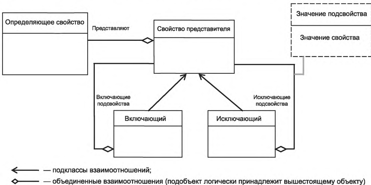
Рисунок 8 — Иерархия вычисления определяющих свойств
