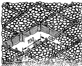
РИС. 7. КАМЕННАЯ НАБРОСКА В ЛЕТНЕВЫЕ КЛЕТКИ
