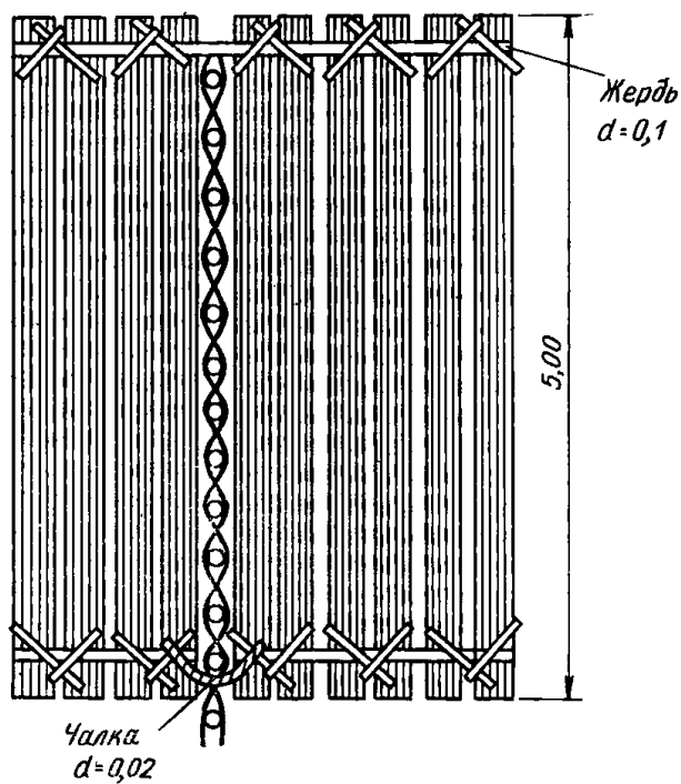
РИС. 13. ПЛОТ ДЛЯ УСТРОЙСТВА ПЛЕТНЯ
