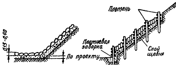
РИС. 8. МОЩЕНИЕ КАМНЕМ
