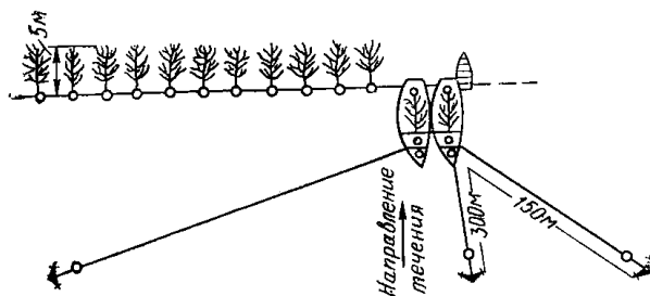
РИС. 21. УСТРОЙСТВО ЗА- ВЕС НА КОЛЬЯХ (СХЕМА ОРГАНИЗАЦИИ РАБОТ)
