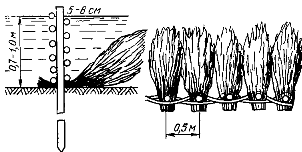
РИС. 16. ОДНОРЯДНЫЙ ПЛЕТЕНЬ С ДОННОЙ ХВОРОСТАНОЙ ВЫСТИЛКОЙ
