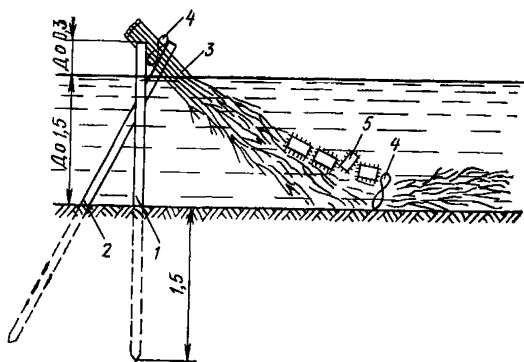
РИС. 12. ПОЛУЗАПРУДА ИЗ МЕТЛОВЫХ ЩИТОВ
