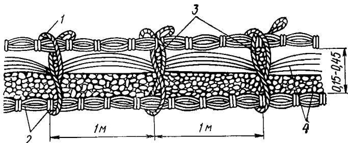
РИС. 10. ХВОСТЯНОЙ ТЮФЯК
