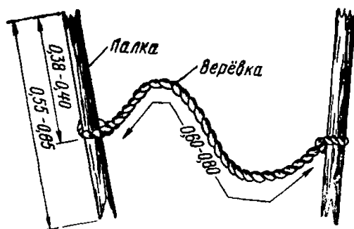
РИС. 24. ВЕРЕВОЧНЫЙ СЖИМ
