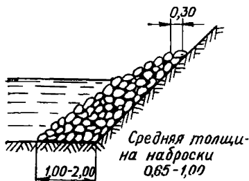
РИС. 6. КАМЕННАЯ НАБРОСКА
