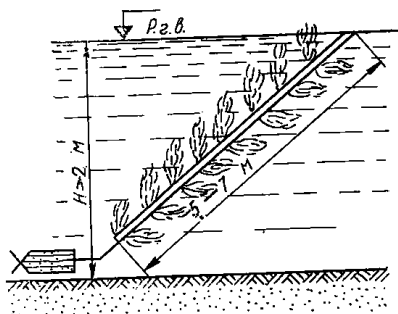
РИС. 19. УСТРОЙСТВО ВЕТВИСТЫХ ЗАГРЯЖДЕ- НИЙ НА ЯКОРЯХ
