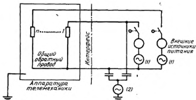
а) схема для активных двоичных входных сигналов
