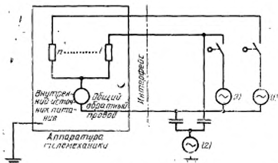
б) схема для пассивных двоичных входных сигналов
