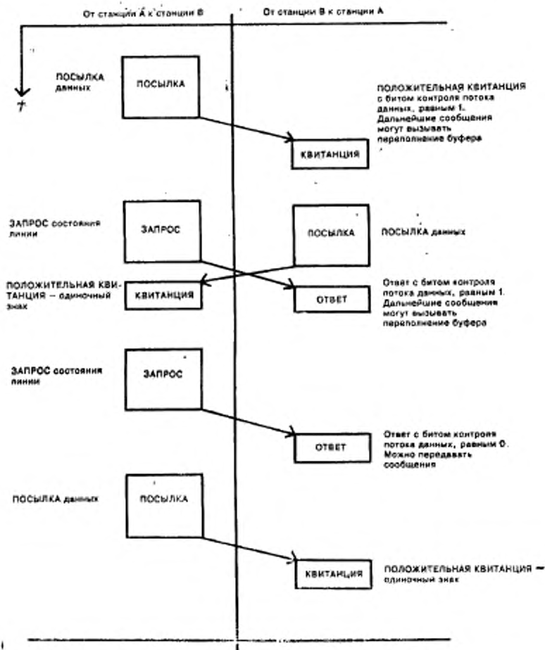
Рисунок 12 — Балансные процедуры передачи. Контроль потока данных
