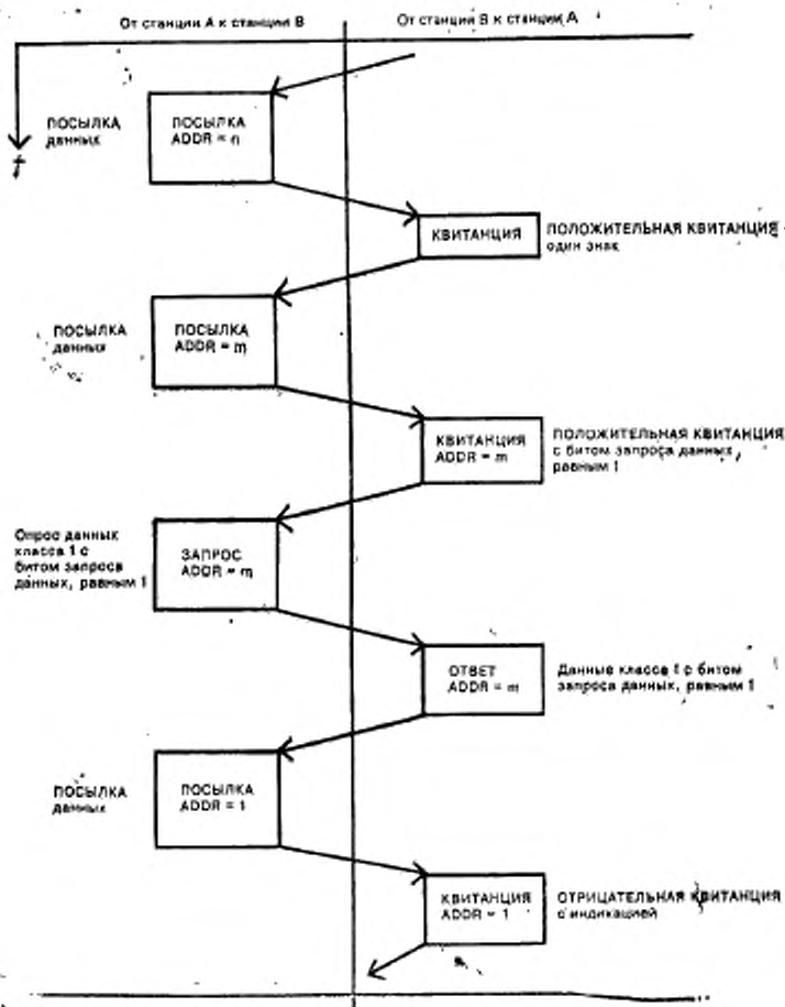
Рисунок 3 — Небалансные процедуры передачи, неискаженные процедуры ПОСЫЛКА/ПОДТВЕРЖДЕНИЕ
