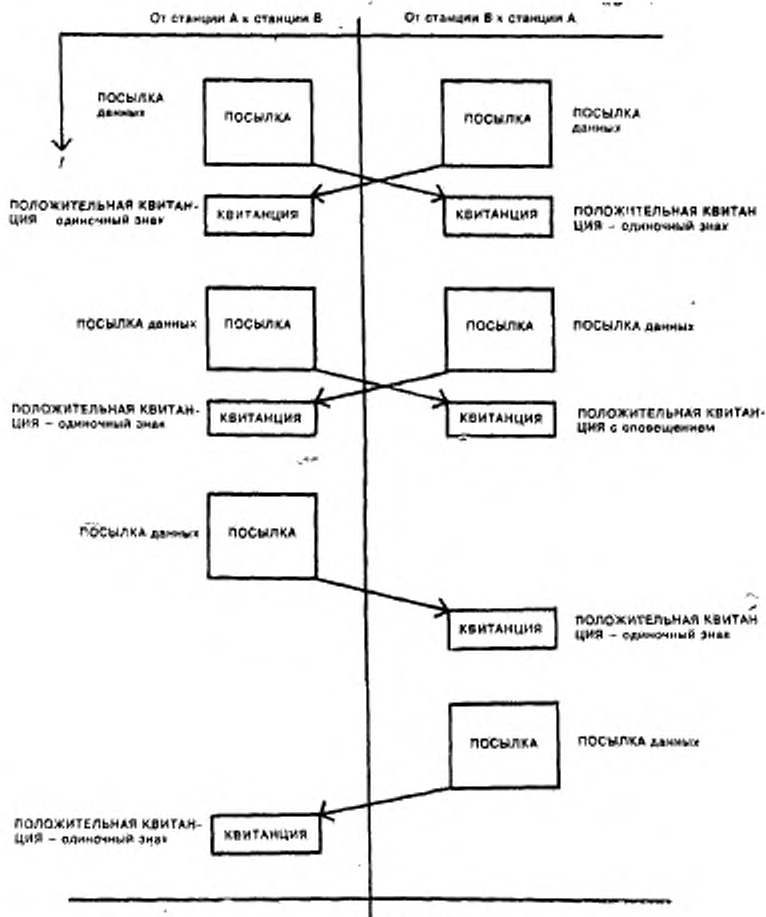
Рисунок 11 — Балансные процедуры передачи. Неискаженные процедуры ПОСЫЛКА/ПОДТВЕРЖДЕНИЕ
