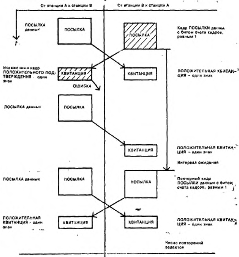
Рисунок 15 — Базисные процедуры передачи. Искорженный кадр ПОДТВЕРЖДЕНИЯ
