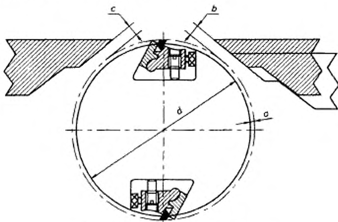
Рисунок 101 — Ножевой блок
