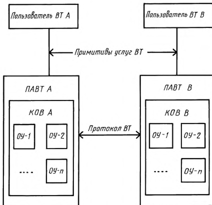
Рисунок 2 — Объекты управления в модели протокола ВТ
