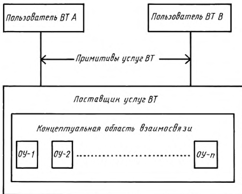
Рисунок 1 — Объекты управления в модели услуг ВТ
