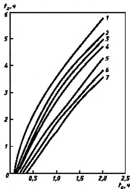
Рисунок Л.8 — Зависимость эквивалентной продолжительности пожара t_{\text{экв}} от характерной продолжительности объемного пожара t_{\text{н}} для железобетонных несущих стен
