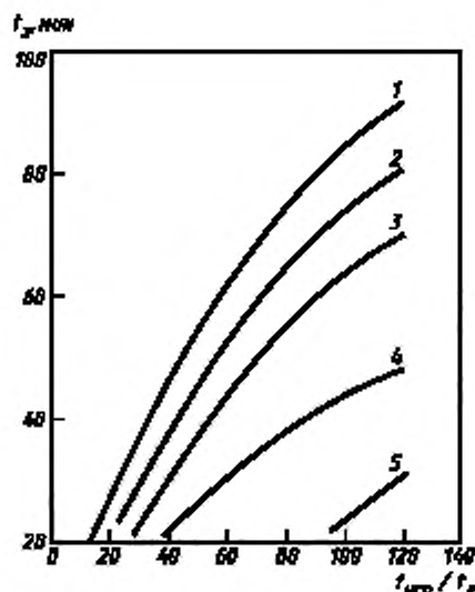
1 — H/\sqrt{F} = 1,2 ; 2 — H/\sqrt{F} = 1,5 ; 3 — H/\sqrt{F} = 1,8 ; 4 — H/\sqrt{F} = 2,2 ; 5 — H/\sqrt{F} = 2,4
