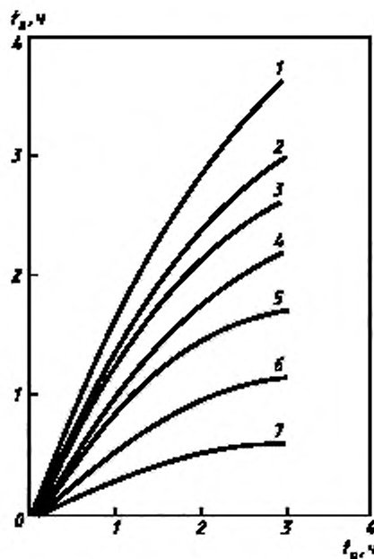
Рисунок Л.7 — Зависимость эквивалентной продолжительности пожара t_{\text{экв}} от характерной продолжительности пожара t_{\text{н}} для огнезащищенных металлических и железобетонных конструкций перекрытия
