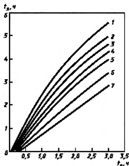
Рисунок Л.9 — Зависимость эквивалентной продолжительности пожара t_{\text{экв}} от характерного времени объемного пожара t_{\text{н}} для центрально сжатых железобетонных колонн
