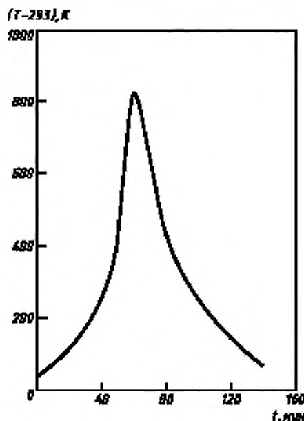
Рисунок К.1 — Изменение среднееобъемной температуры по времени с учетом начальной стадии пожара
