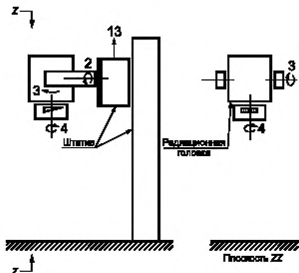
Рисунок 1 — Ротационный ШТАТИВ
