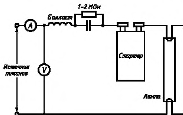
Рисунок 7 — Схема испытания стартеров на зажигание
