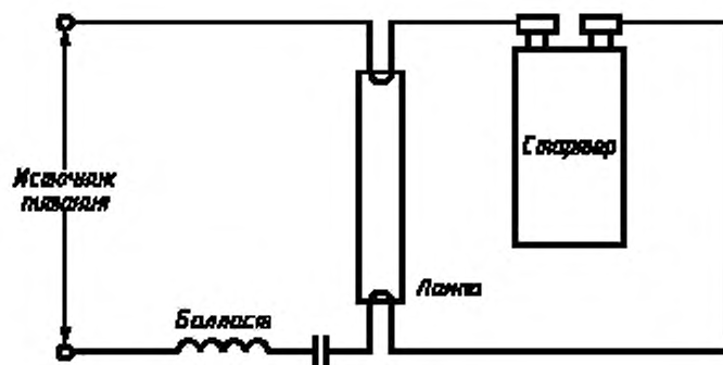
Рисунок 10 — Схема испытания стартеров на долговечность
