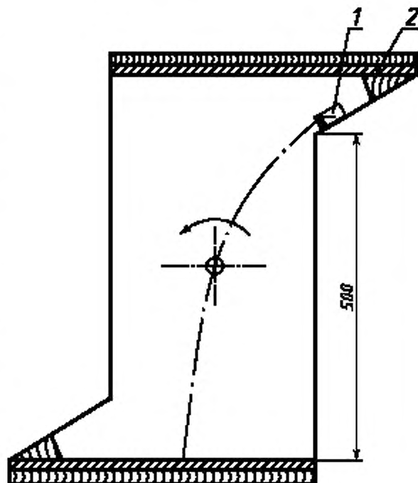
1 — стартер, 2 — стальная пластина
