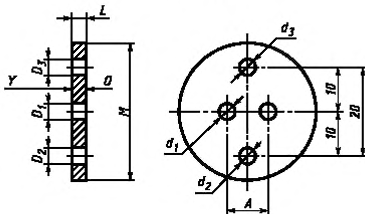
Рисунок 1 — Размеры стартеров
