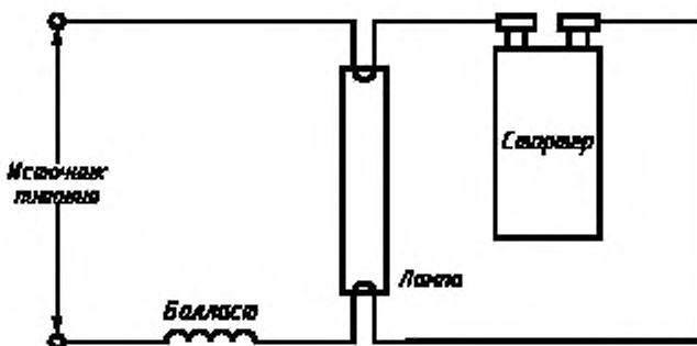
Рисунок 9 — Схема испытания стартеров на долговечность
