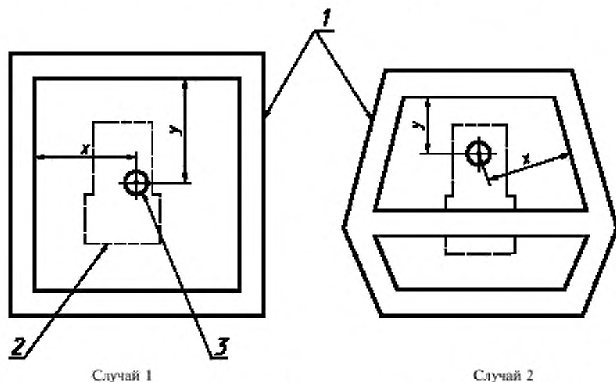
Рисунок 2 — Точки приложения удара 1 — главный верхний горизонтальный элемент; 2 — вертикальная проекция зоны ограничения деформации; 3 — конус стандартного предмета
