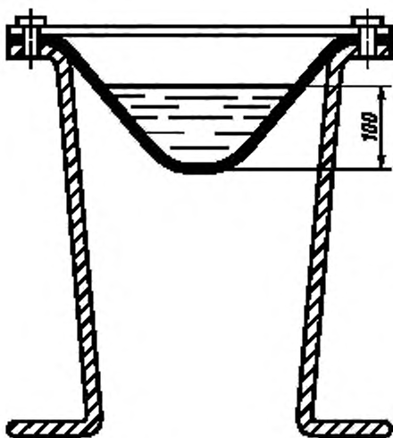
Рисунок 4 — Приспособление для определения водопроницаемости методом кошеля
