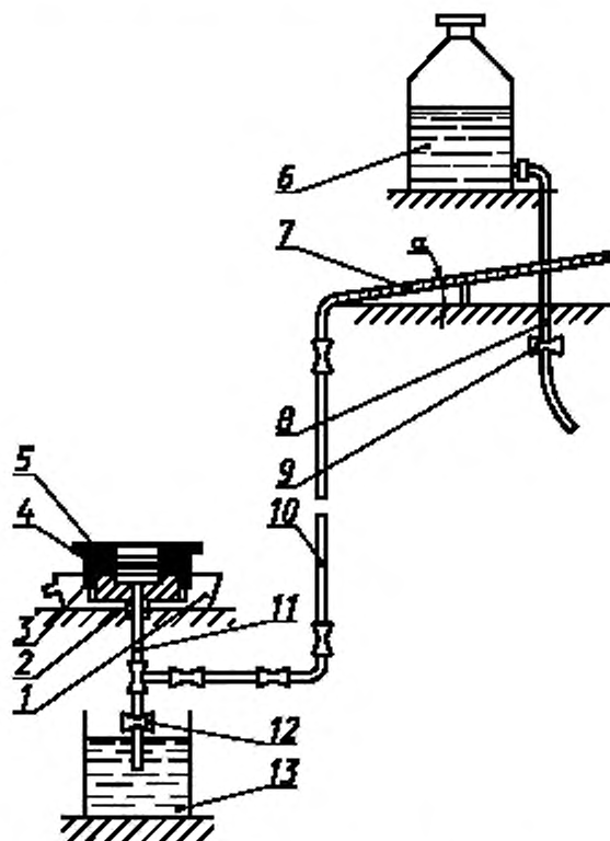
1 — ванна; 2 — полая камера; 3 — крышка; 4 — резиновая уплотняющая прокладка; 5 — металлическая прокладка; 6 — сосуд с тубусом для воды; 7 — стеклянная градуированная трубка; 8, 11 — резиновые трубки; 9, 12 — зажимы на трубках; 10 — стеклянная трубка; 13 — бачок для слива воды
