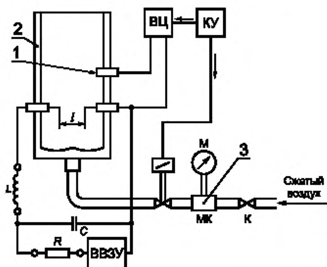
ВЦ — вспомогательная цепь; C — испытательный конденсатор; КУ — контрольное устройство; ВВЗУ — зарядное устройство; M — манометр; L — индуктивность; МК — магнитный клапан; R — зарядное сопротивление; К — запорный клапан; I — основной межэлектродный промежуток; 1 — вспомогательный электрод; 2 — трубка Хартмана; 3 — резервуар сжатого воздуха
