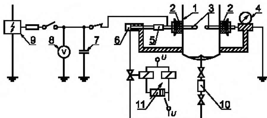
1 — камера для воспламенения, трубка Хартмана с открытой верхней частью; 2 — пробки из ПТФЭ; 3 — электроды; 4 — микрометрический винт; 5 — изоляционный отрезок трубы из ПТФЭ; 6 — пневматический поршень двойного действия; 7 — конденсатор; 8 — электростатический вольтметр; 9 — генератор высокого напряжения (5–10 кВ); 10 — камера высокого давления; 11 — таймер
