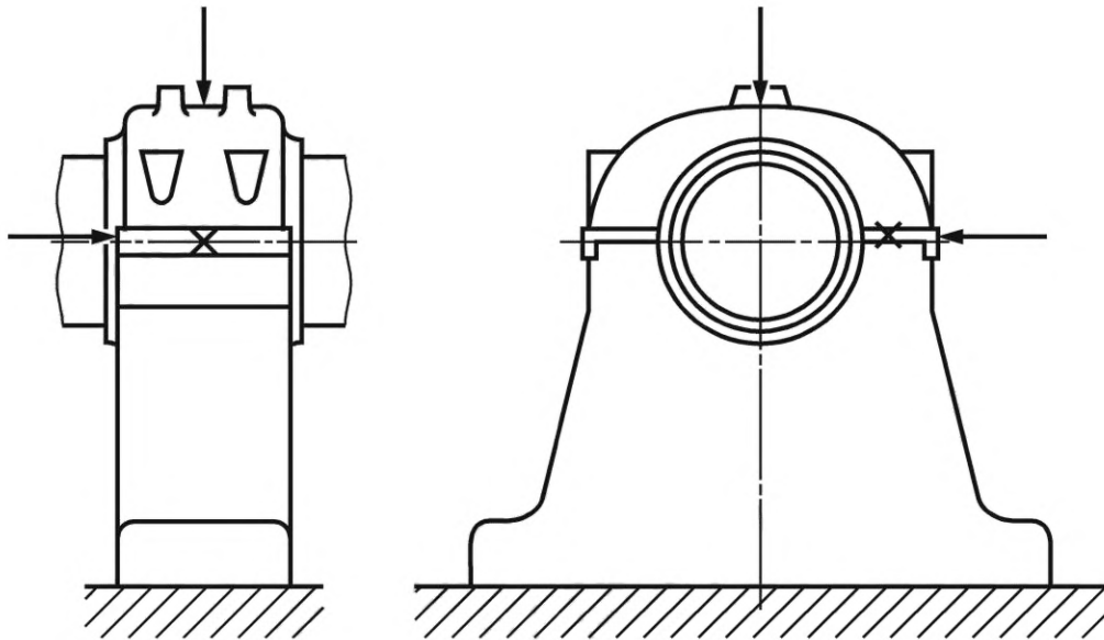
Рисунок 1 — Точки измерений на опорах/крышках подшипников
