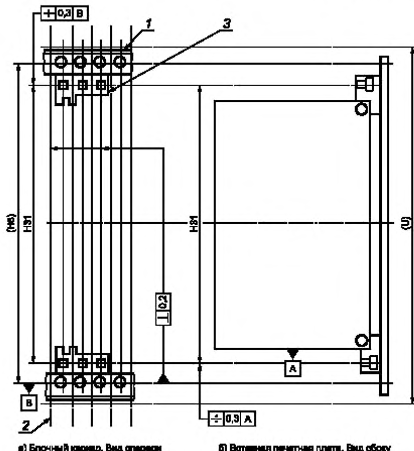
а) Блочный каркас. Вид спереди
