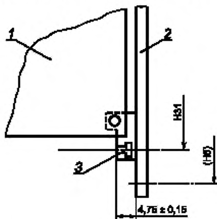
1 — печатная плата, 2 — лицевая панель вставного блока; 3 — размеры места для установки опорной части ключа, см. раздел 5
