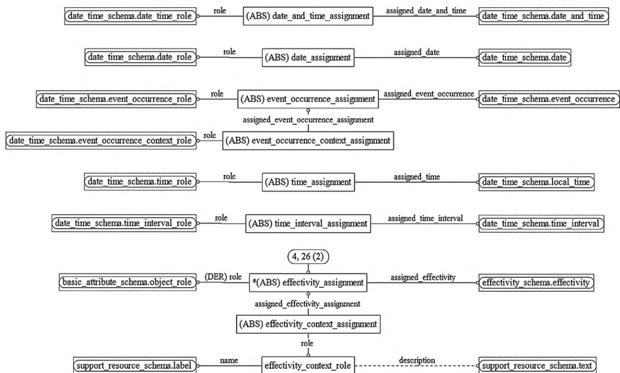
Рисунок D.36 — EXPRESS-G диаграмма схемы management_resources_schema (диаграмма 4 из 9)
