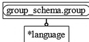
Рисунок D.30 — EXPRESS-G диаграмма схемы language_schema (диаграмма 2 из 2)
