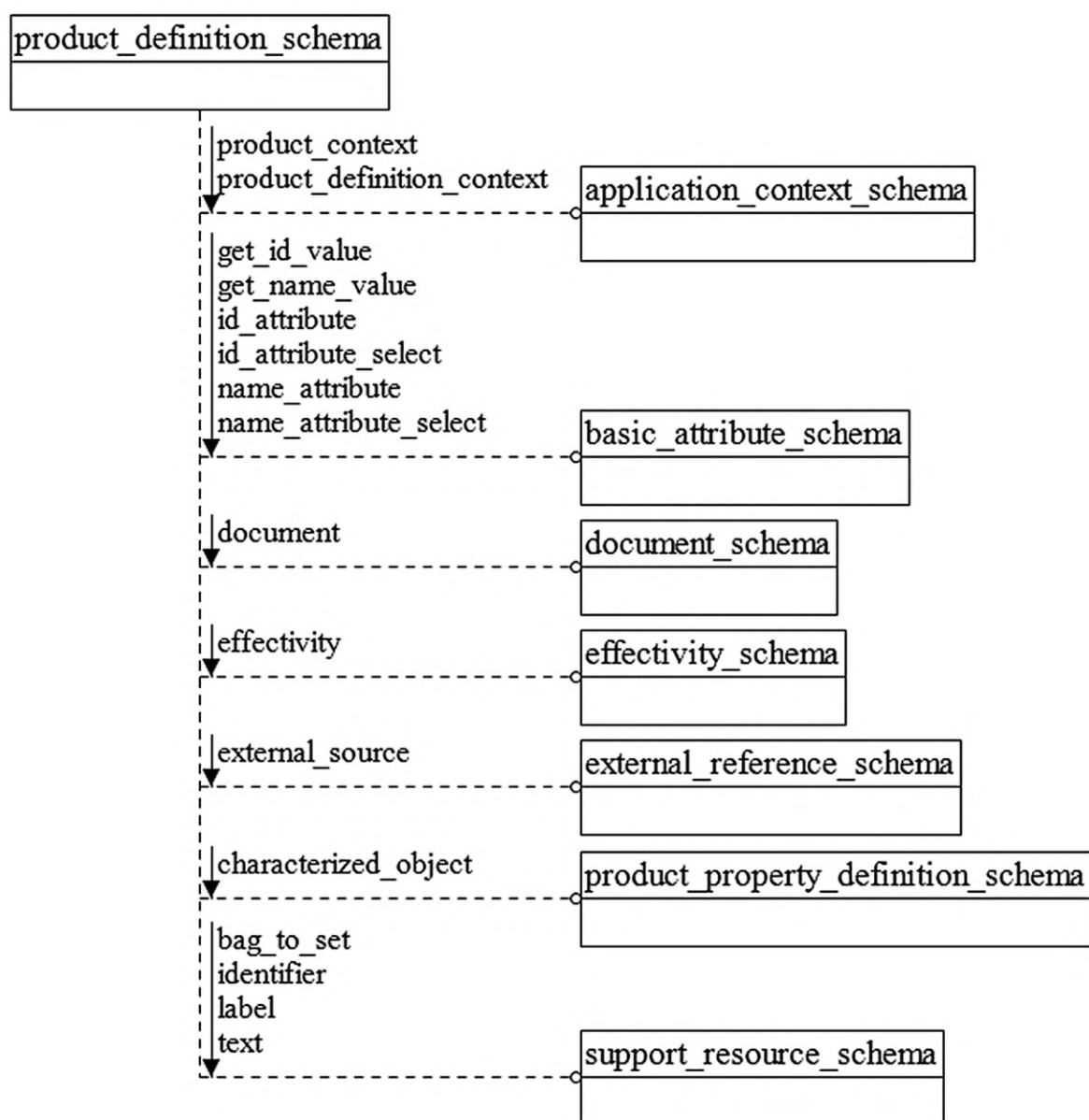
Рисунок D.51 — EXPRESS-G диаграмма схемы product_definition_schema (диаграмма 1 из 3)
