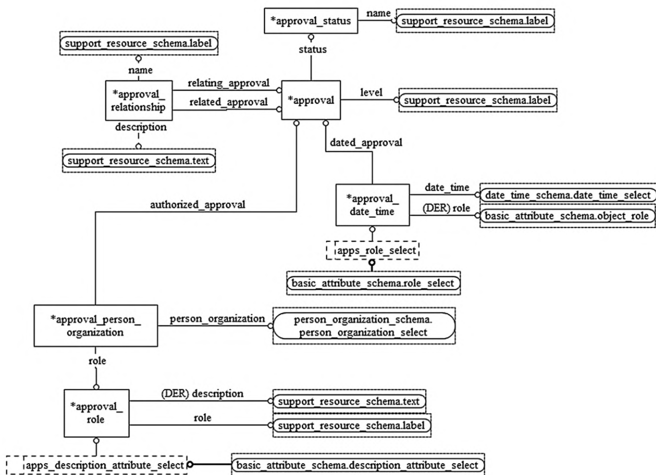
Рисунок D.6 — EXPRESS-G диаграмма схемы approval_schema (диаграмма 2 из 2)
