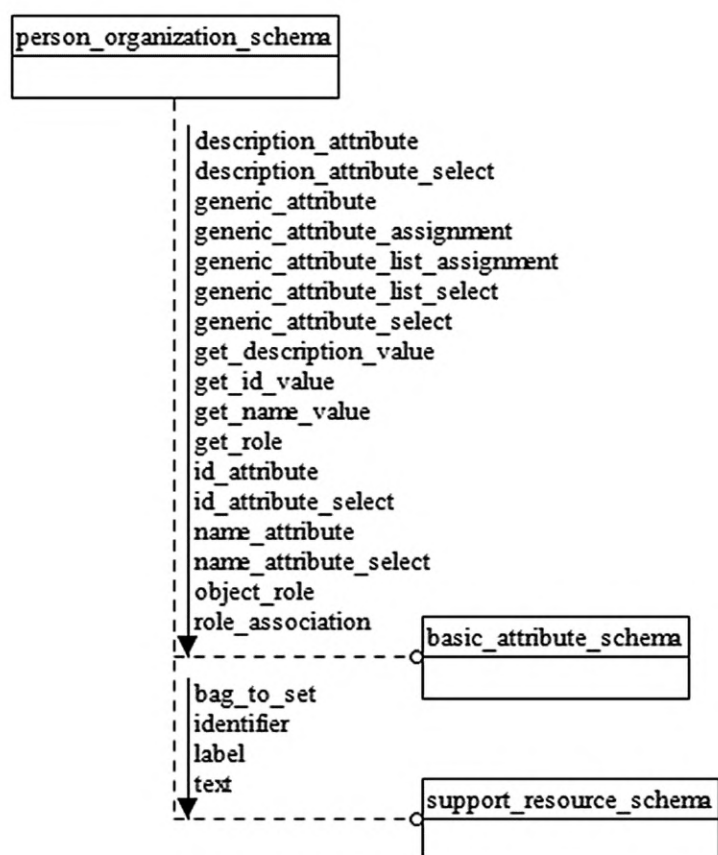
Рисунок D.47 — EXPRESS-G диаграмма схемы person_organization_schema (диаграмма 1 из 4)
