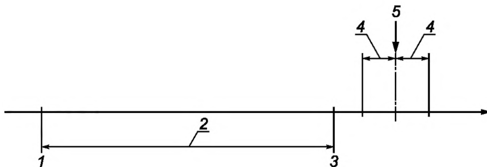
1 — нижний предел установленного диапазона значений; 2 — диапазон допустимых значений; 3 — верхний предел установленного диапазона значений; 4 — неопределенность измерения U ; 5 — измеренное значение
